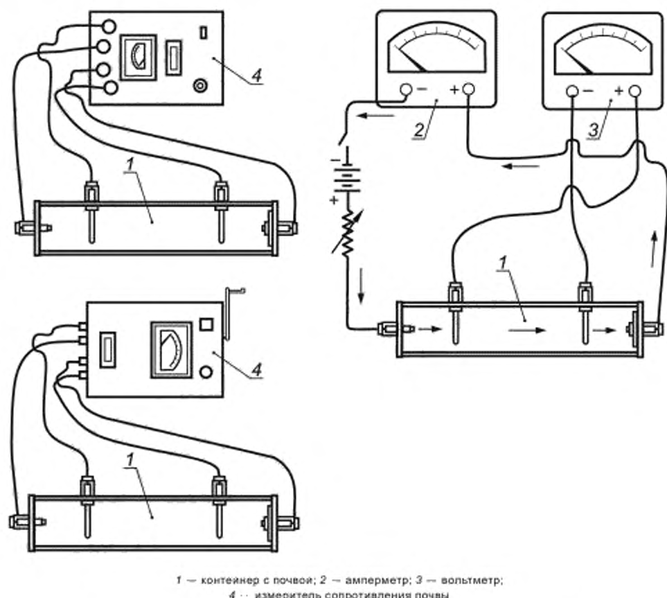
Рисунок 1 — Устройство контейнера с четырьмя электродами и с почвой
