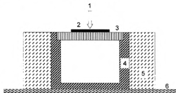
1 – усилие; 2 – круглая стальная плита; 3 – съемная крышка; 4 – оболочка; 5 – бетонная форма; 6 – жесткое основание
