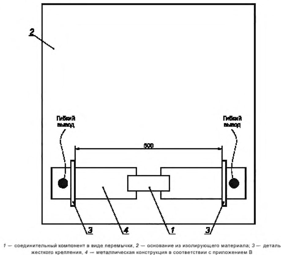
Рисунок 3 — Пример соединения перемычкой
