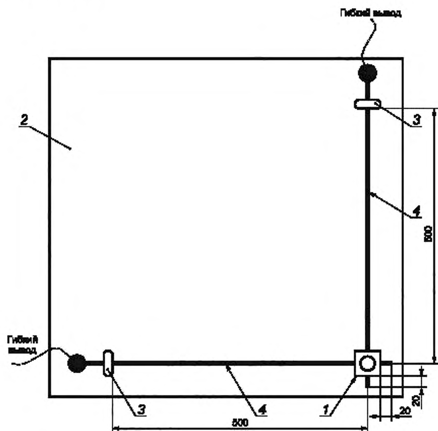
Рисунок 1 — Пример перекрестного соединения
