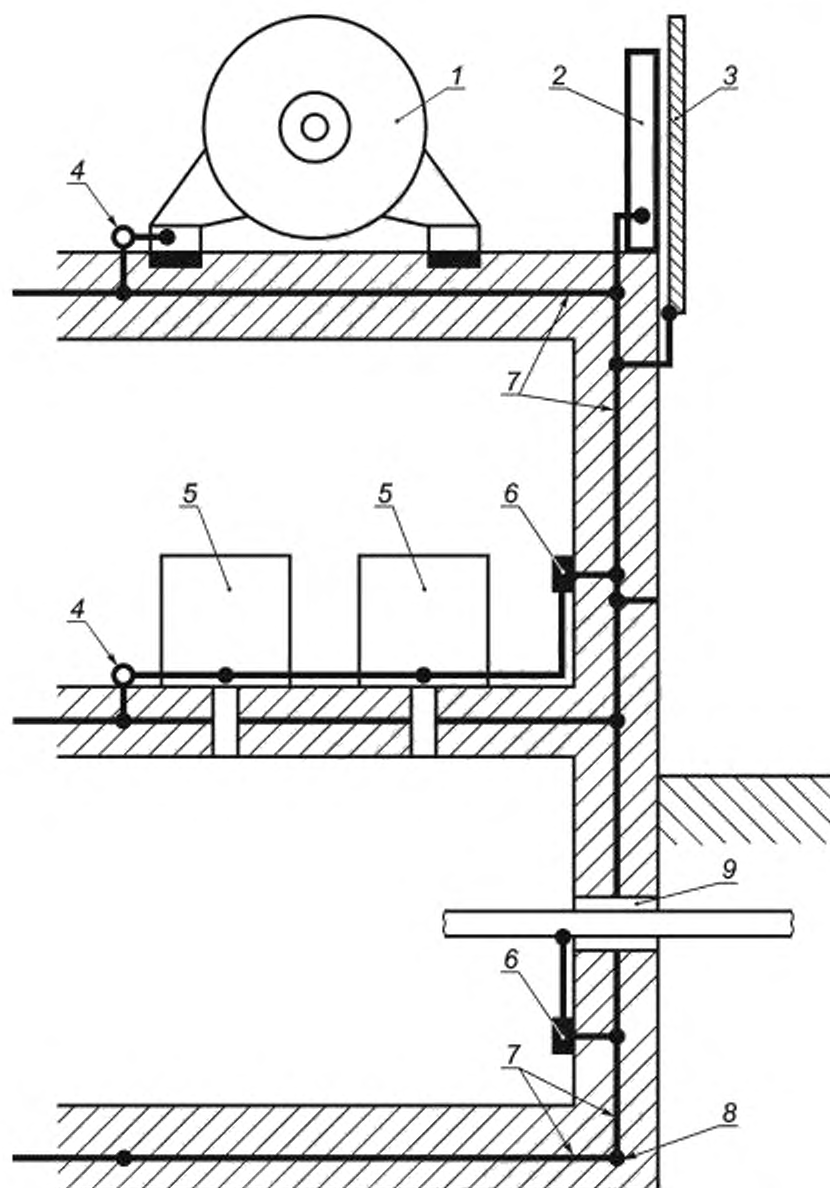
1 — электрическое силовое оборудование; 2 — стальная балка; 3 — металлическое покрытие фасада; 4 — точка присоединения; 5 — электрический или электронный виды оборудования; 6 — шина уравнивания потенциалов; 7 — стальная арматура железобетона (с наложенными проводниками сетки); 8 — фундаментный заземлитель; 9 — общий ввод различных коммуникаций
