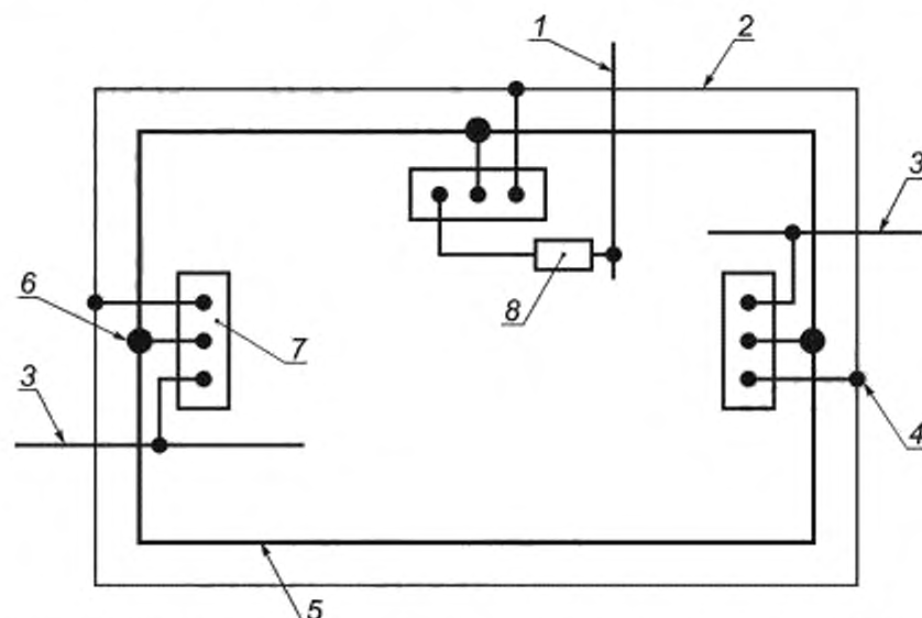
1 — линия электроснабжения или линия связи; 2 — внешний горизонтальный кольцевой проводник (выше поверхности грунта); 3 — внешняя проводящая часть; 4 — присоединение к токопроводу; 5 — стальная железобетонная арматура в стене; 6 — точка уравнивания потенциалов с арматурой железобетона; 7 — шина уравнивания потенциалов; 8 — устройство защиты от перенапряжений
