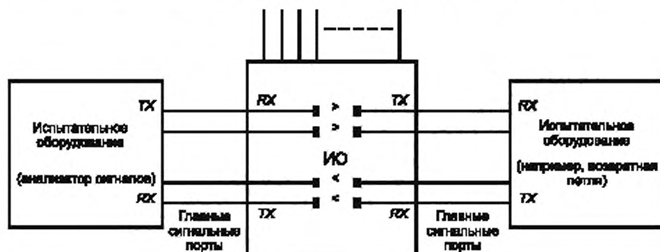
Рисунок 2 — Схема испытательной конфигурации
