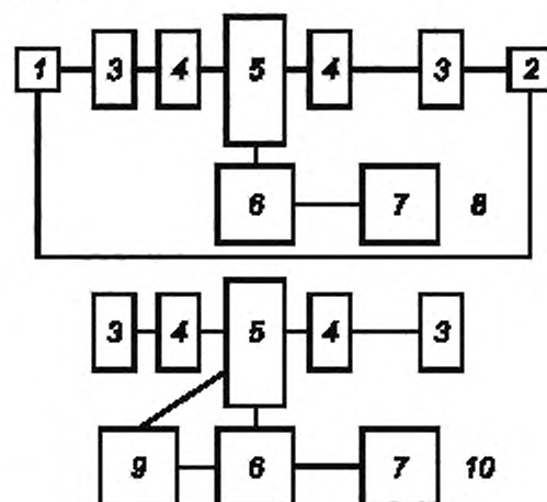
1 — имитатор трафика А; 2 — имитатор трафика В; 3 — блок цифровых линий; 4 — группа магистральных линий; 5 — коммутационная сеть; 6 — центральный процессор; 7 — контрольный блок; 8 — испытываемое оборудование А; 9 — имитатор испытательной нагрузки; 10 — испытываемое оборудование В
