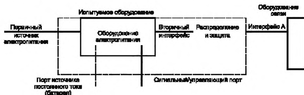
Рисунок 4 — Общая схема источника электропитания и его портов
