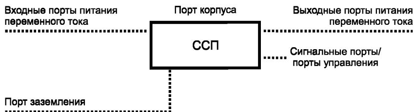
Рисунок 1 — Примеры портов
