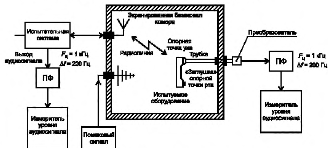
Рисунок 1 — Схема прохождения сигнала при испытаниях
