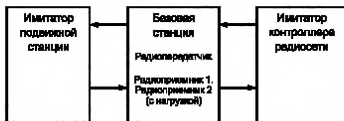
Рисунок 1 — Схема испытаний на помехоустойчивость базовой станции
