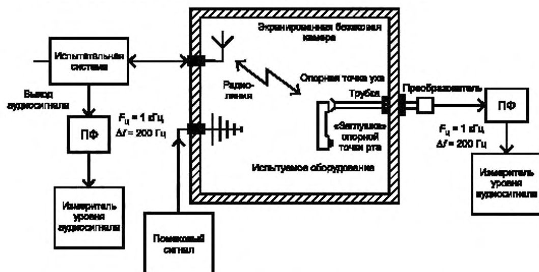
ПФ — полосовой фильтр; F_{ц} — центральная частота полосы пропускания полосового фильтра; \Delta f — полоса пропускания фильтра
