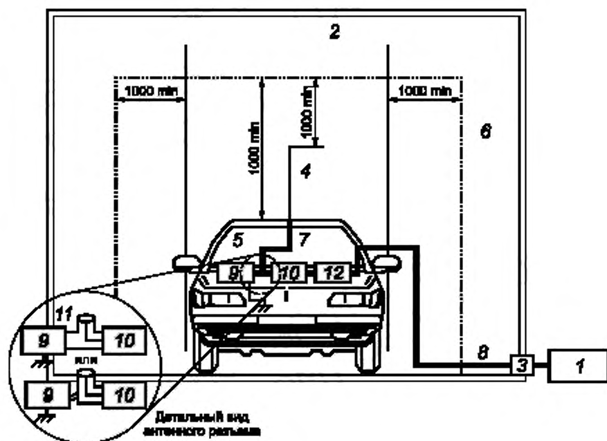
1 — измерительное устройство, 2 — БЭК; 3 — проходной разъем, 4 — антенна (см. 5.1); 5 — транспортное средство, 6 — типовой поглощающий материал; 7 — антенный коаксиальный кабель, 8 — коаксиальный кабель высокого качества с двойным экранированием (50 Ом); 9 — корпус бортовой радиосистемы; 10 — схема согласования (если требуется); 11 — модифицированный коаксиальный разъем (T-типа), 12 — схема изоляции от заземления в полосе АМ вещания (если требуется)
