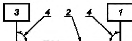
1 — ИО, 2 — испытуемые провода; 3 — имитатор нагрузки; 4 — угол (90^{+45}_0)^\circ
