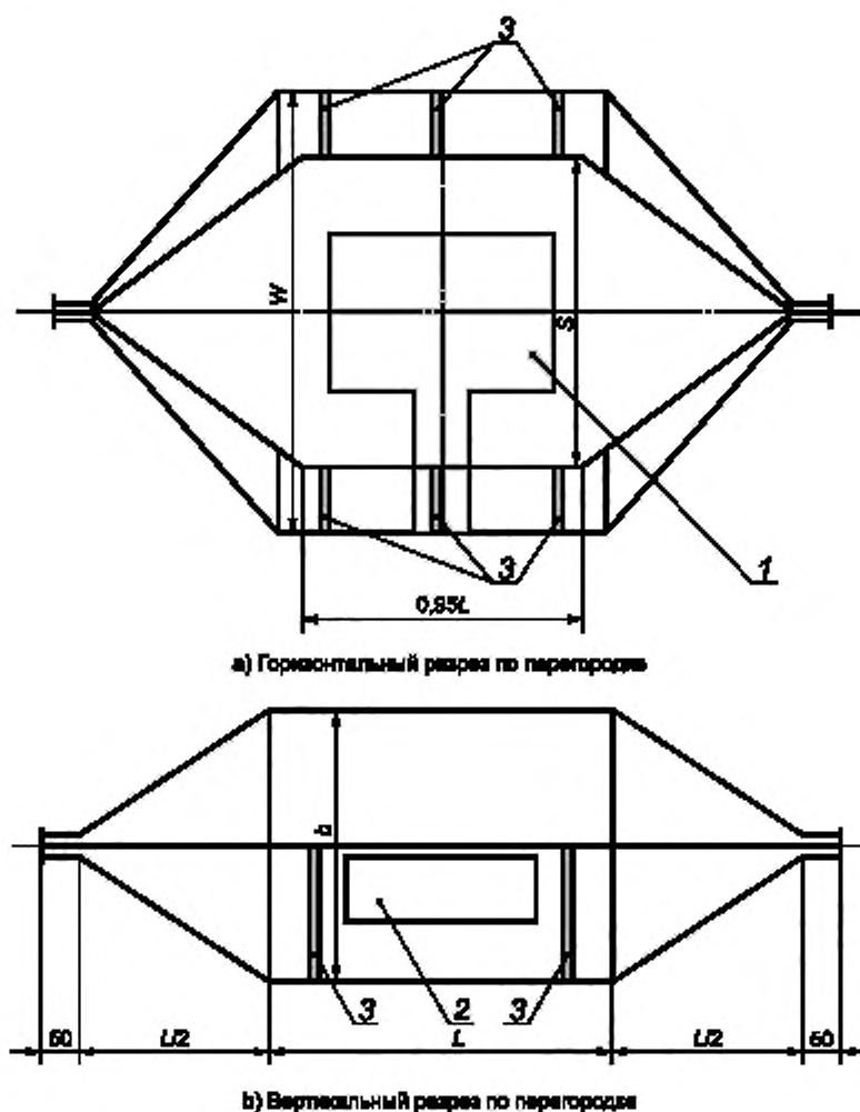
Рисунок F.1 — ТЕМ-камера
