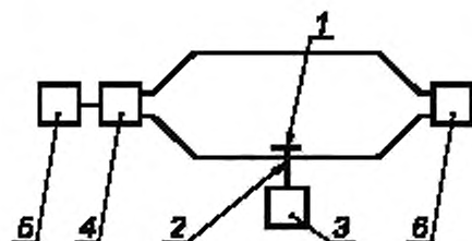
Рисунок F.1 — Структурная схема калибровки ТЕМ-установки
