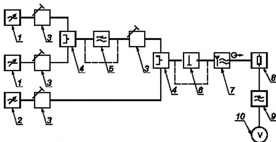
1 — генератор мешающего сигнала (G1); 2 — генератор полезного сигнала (G2); 3 — аттенюаторы; 4 — схема связи; 5 — фильтр нижних частот 1) ; 6 — схема согласования и/или симметрирования; 7 — испытуемое оборудование 2) ; 8 — нагрузочный резистор; 9 — фильтр нижних частот (см. приложение В); 10 — вольтметр звуковой частоты (со схемой взвешивания в соответствии с [4])
