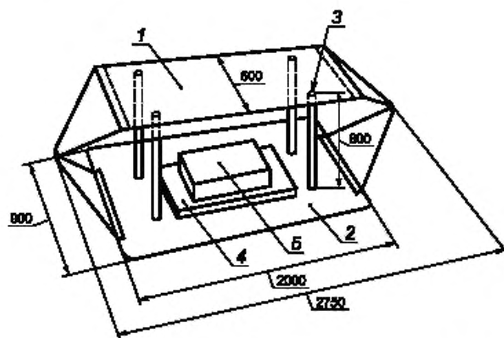
1 — металлическая верхняя пластина площадью 2×0,8 м, параллельная пластине основания; 2 — металлическая пластина основания площадью 2×0,9 м; 3 — пластмассовые распорки (высотой 0,8 м — 4 шт.); 4 — неметаллическая подставка; 5 — испытуемое ТС
