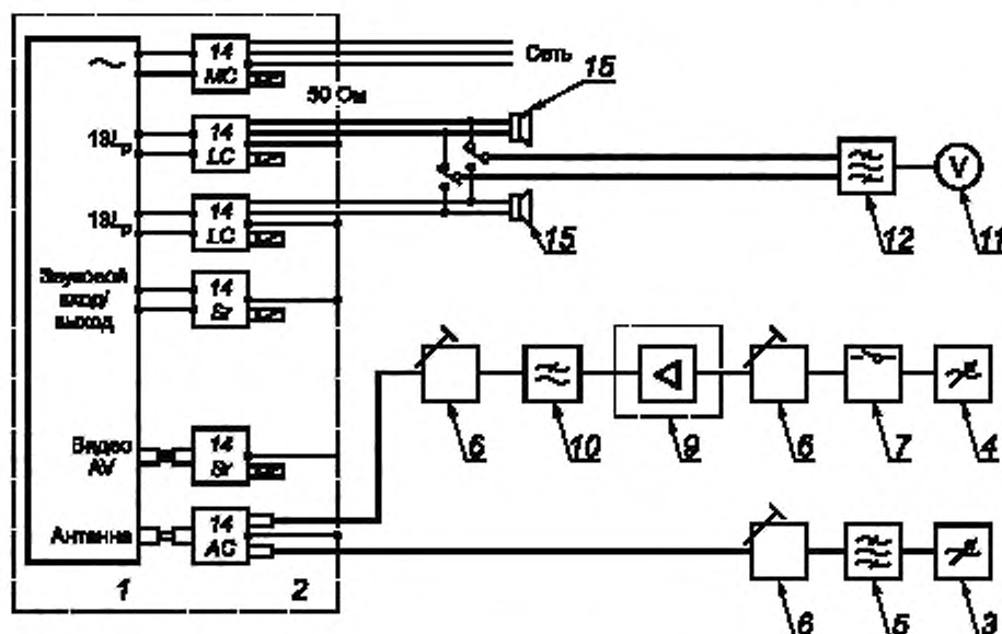
1 — испытуемое оборудование; 2 — металлическая пластина площадью 2 \times 1 м; 3 — генератор полезного сигнала (G1); 4 — генератор мешающего сигнала (G2); 5 — канальный фильтр F_c ; 6 — аттенюаторы T_1, T_2, T_3 ; 7 — переключатель (коммутатор) S1; 8 — усилитель A_m ; 9 — экранированный контейнер S_p ; 10 — фильтр нижних частот F_l ; 11 — вольтметр звуковой частоты V ; 12 — полосовой фильтр 0,5—3 кГц (см. приложение В); 13 — зажимы громкоговорителя L_p ; 14 — блоки УСР типов MC, LC, Sr, AC (см. приложение С); 15 — эквивалент нагрузки, имитирующий номинальное полное сопротивление громкоговорителя
