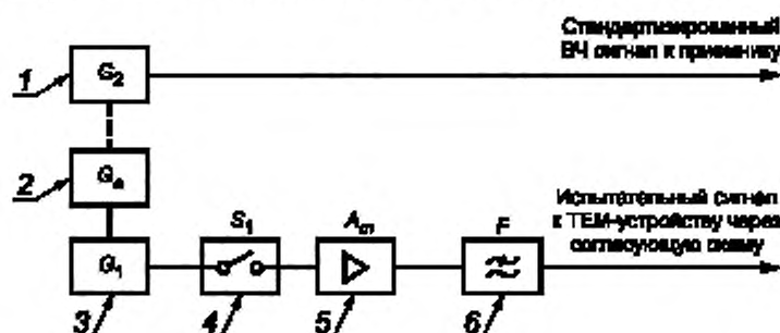
Рисунок 7 — Структурная схема измерения параметров помехоустойчивости радиовещательных приемников по отношению к электромагнитному полю
