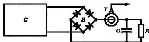
G — испытательный генератор провалов напряжения с переключением при 90^\circ и 270^\circ ; T — токосъемник; B — выпрямительный мост; R — резистор сопротивлением не более 10 кОм и не менее 100 Ом; C — электролитический конденсатор емкостью 1700 мкФ \pm 20\%
