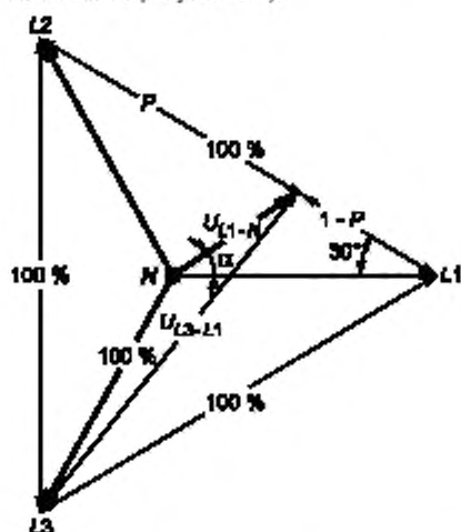
Рисунок В.2 — Векторы напряжений при провале напряжения «фаза — фаза»: допустимый метод 1
