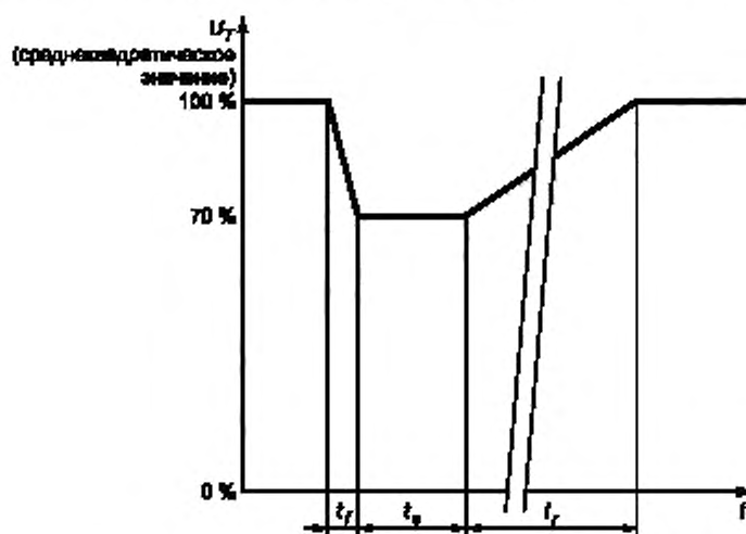
Рисунок 2 — Зависимость изменения напряжения от времени
