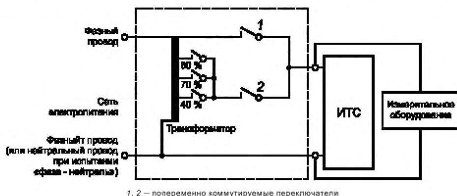
Рисунок Г.1 — Пример устройства ИГ для испытаний при воздействии провалов и кратковременных прерываний напряжения с использованием регулируемого трансформатора и переключателей
