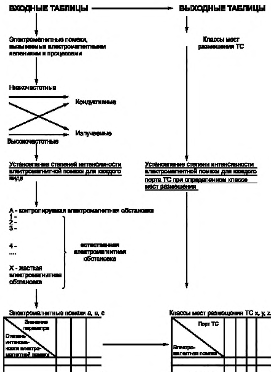
Рисунок 1 — Принципы классификации электромагнитной обстановки
