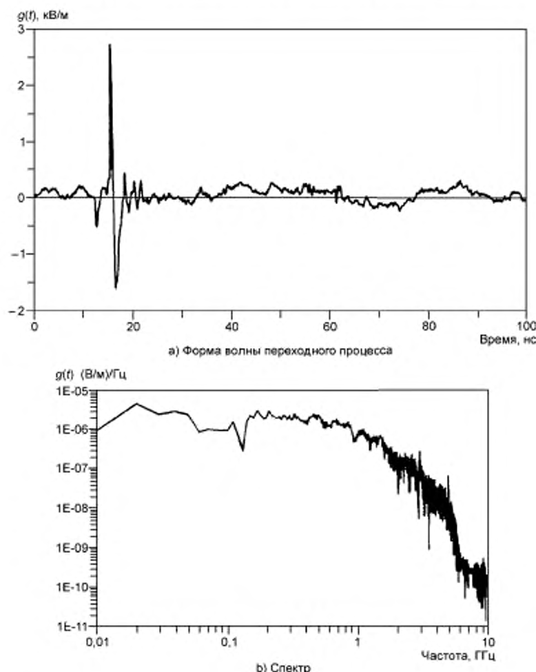
Рисунок 3 — Пример электромагнитного воздействия большой мощности на основе сверхширокополосного переходного процесса (форма волны и спектр)
