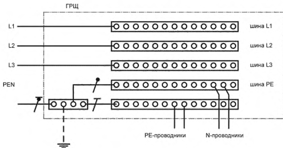
Рисунок 54.1с — Пример 3 ГРЩ — Главный распределительный щит
