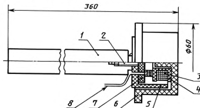
Локальный индукционный преобразователь ИП-1
