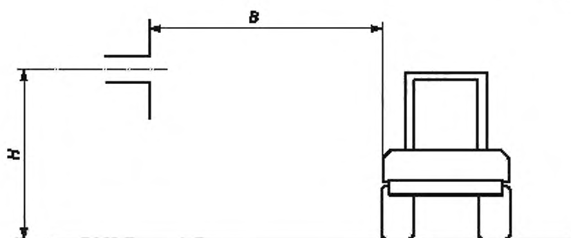
а) Расположение дипольной антенны для измерения излучения с вертикальной поляризацией
