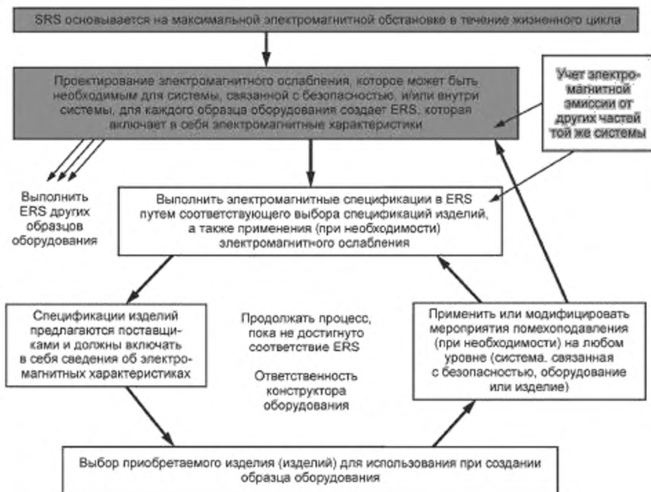
Рисунок D.2 — Процесс достижения электромагнитной спецификации в SRS при использовании коммерчески доступных изделий
