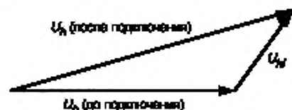
Рисунок 3 — Иллюстрация вектора эмиссии U_{hi} и его вклада в измеряемый вектор гармоник в точке оценки
