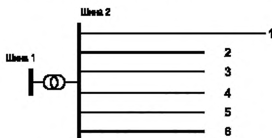
Рисунок В.1 — Пример системы распределения СН, включающей в себя трансформатор СН и фидеры 1—6
