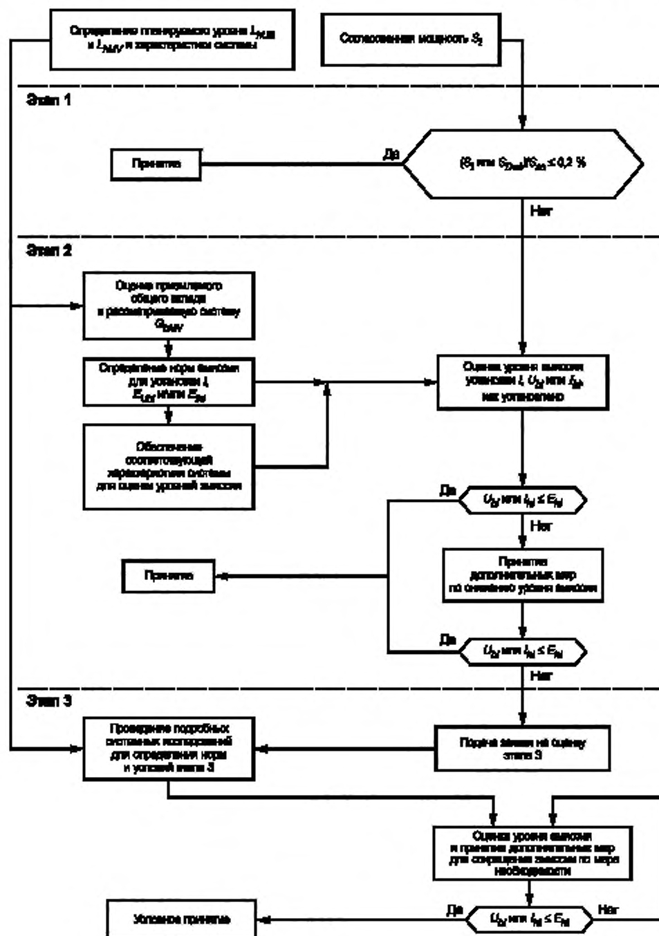
Рисунок 5 — Схема процедуры оценки при среднем напряжении
