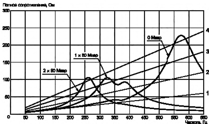
Рисунок D.2 — Гармоническое полное сопротивление в узле 1
