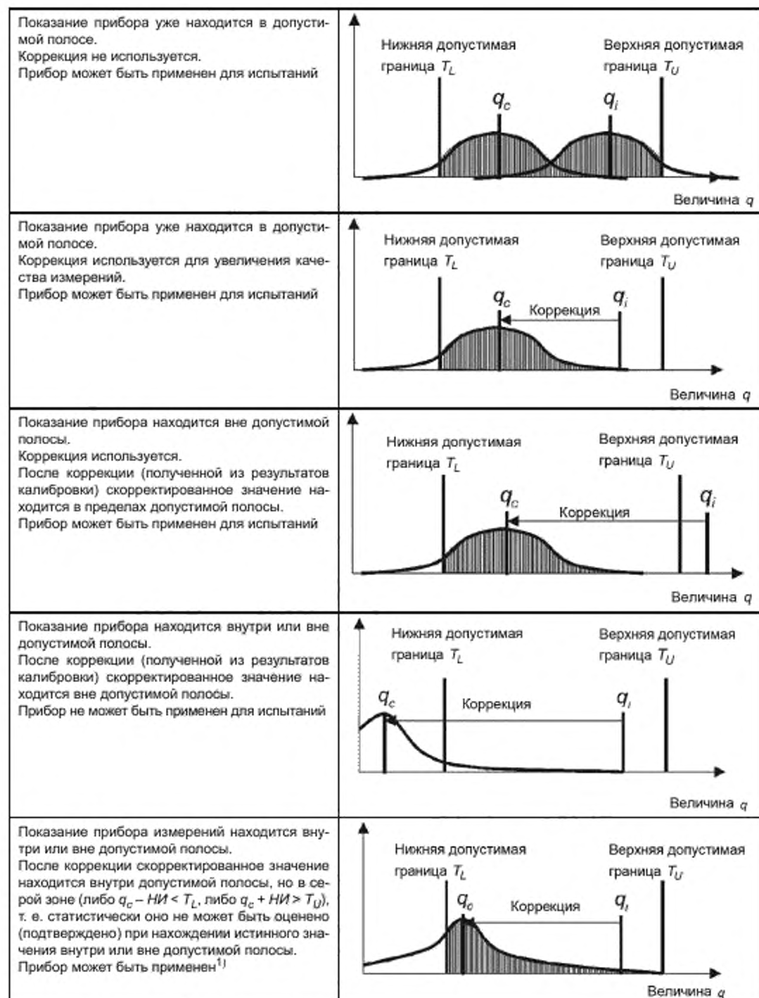
Рисунок 17, лист 1 — Ситуации, показывающие, когда и как средство измерений подходит для испытаний или измерений в соответствии с применяемым основополагающим стандартом, устанавливающим допустимые отклонения
