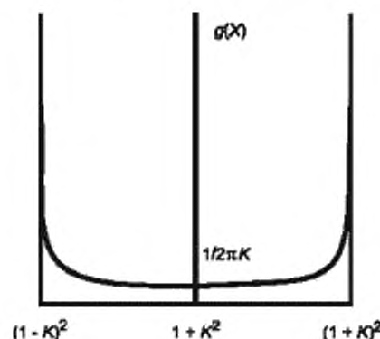
Рисунок 9 — U-образная ФПВ
