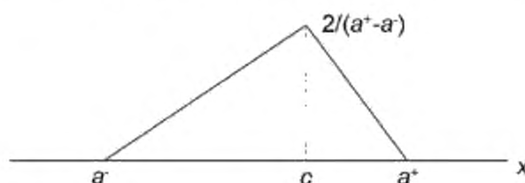
Рисунок 7 — Треугольная ФПВ
