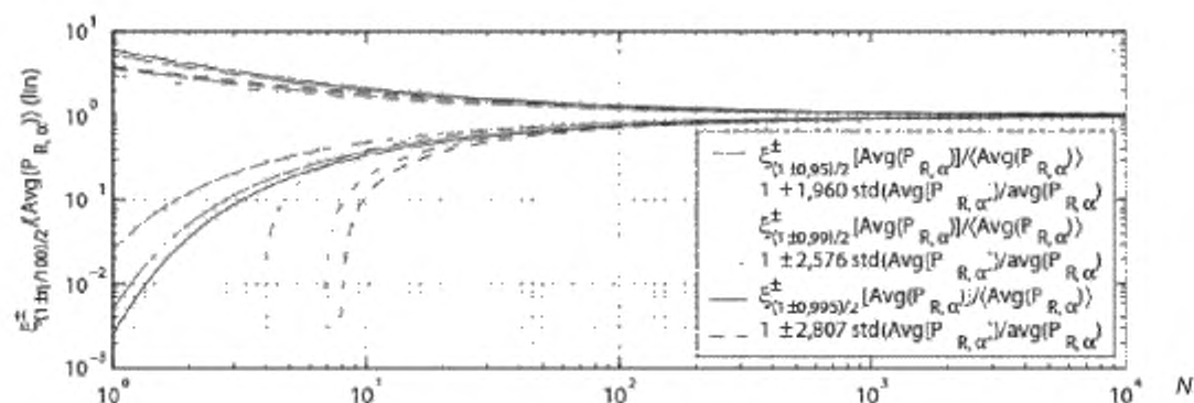
Рисунок 11 — Границы (пределы) доверительных интервалов 95 %, 99 % и 99,5 % для \bar{A} как функции от N для измерений при использовании прямолинейной антенны или одноосного датчика поля
