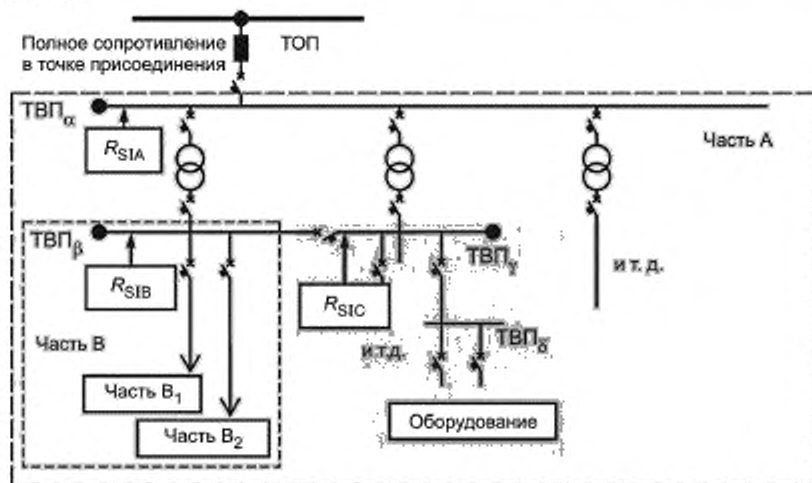
Рисунок В.2 — Топ, ТВП, отношение тока установки и R_{Sl}
