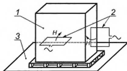
Рисунок 6 — Схема проверки восприимчивости испытуемого оборудования на устойчивость к магнитному полю промышленной частоты методом приближения
