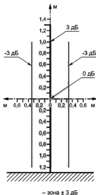
Рисунок В.8 — Зона \pm 3 дБ магнитного поля, создаваемого индукционной катушкой прямоугольной формы (с размерами сторон 1 \times 2,6 м), нижней стороной которой является плоскость заземления, в центральной ортогональной плоскости (компонента, перпендикулярная плоскости катушки)
