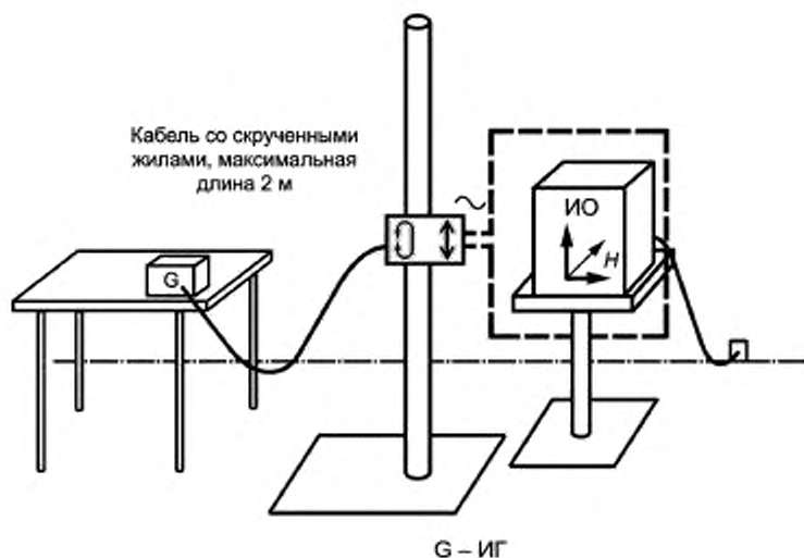
Рисунок 3 — Пример организованного места для испытаний настольного ИО
