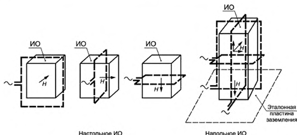
Рисунок 1 — Схема воздействия магнитным полем промышленной частоты на ИО с использованием иммерсионного метода
