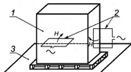
1 — ИО; 2 — индукционная катушка; 3 — эталонная пластина заземления
