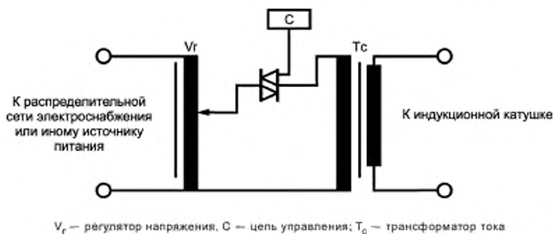
Рисунок 2 — Схема испытательного генератора магнитного поля промышленной частоты
