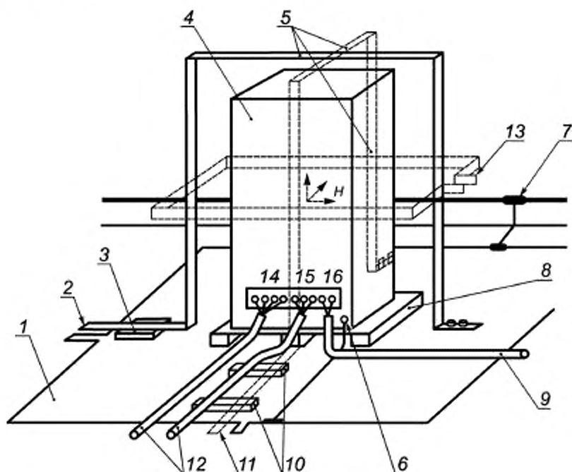
1 — эталонная пластина заземления; 2, 13 — к ИГ; 3, 8, 10 — изоляционная опора; 4 — ИО; 5 — индукционная катушка; 6 — клемма заземления; 7 — соединение плоскости заземления с цепью защитного заземления; 9 — к сети электропитания; 11 — к ИГ; 12 — к источнику сигналов (имитатору); 14 — вводы сигнальной цепи; 15 — вводы коммуникационной линии; 16 — вводы цепи электропитания
