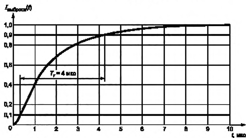
Рисунок Е.11 — Выброс тока (5/320 мкс): длительность переднего фронта T_f
