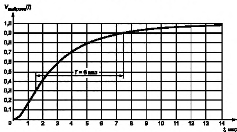
Рисунок E.8 — Выброс напряжения (10/700 мкс): длительность переднего фронта T
