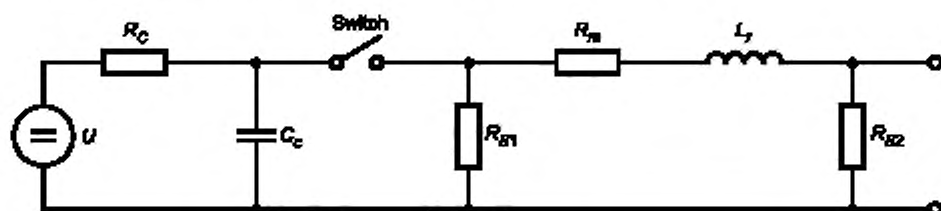
U — источник высокого напряжения; R_C — зарядный резистор; C_C — накопительный конденсатор; R_{S1} — резисторы, формирующие форму импульса; R_m — резистор, соответствующий полному сопротивлению; L_r — индуктивность, формирующая время нарастания; Switch — выключатель
