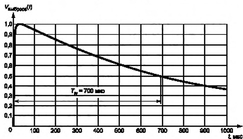
Рисунок E.7 — Выброс напряжения (10/700 мкс): длительность импульса T_w
