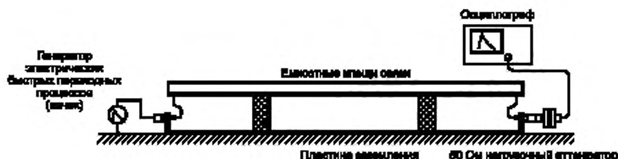
Рисунок 10 — Пример проверки емкостных клещей связи
