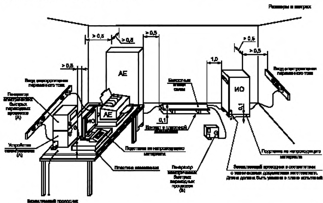
Рисунок 11 — Пример испытательной установки для лабораторных типовых испытаний
