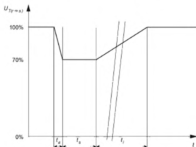
Рисунок 2 — Изменение напряжения
