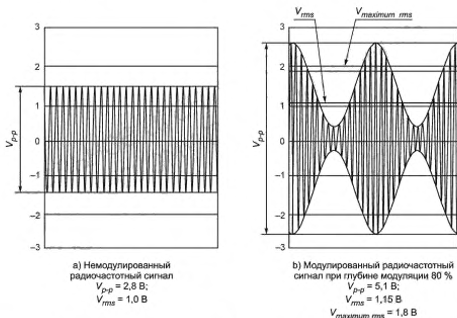
Рисунок 1 — Определение испытательного уровня и формы колебаний на выходе генератора сигналов
