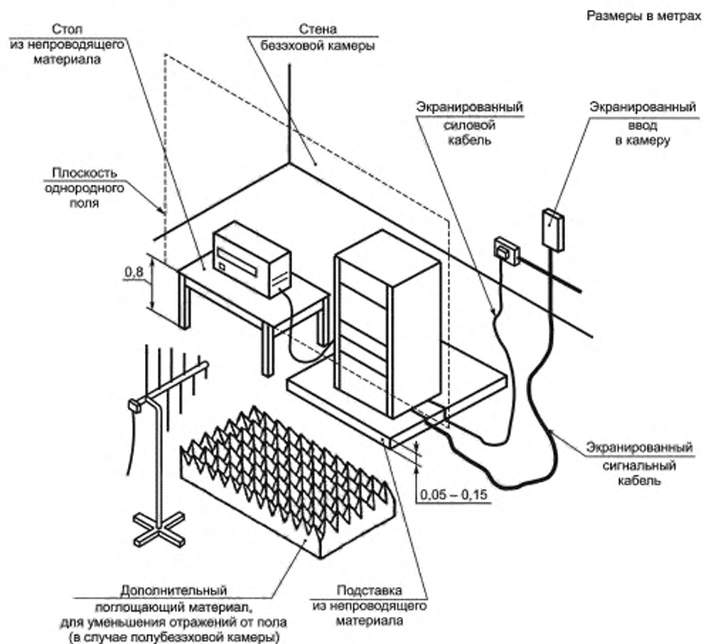
Рисунок 5 — Пример испытательной установки для напольного оборудования
