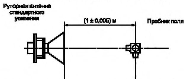
Рисунок 1.10 — Расположение пробника поля при калибровке (вид сверху)
