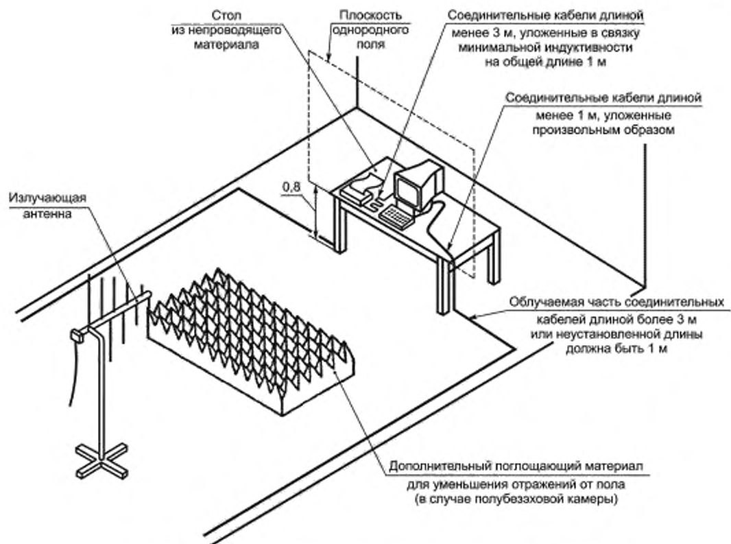
Рисунок 6 — Пример испытательной установки для настольного оборудования
