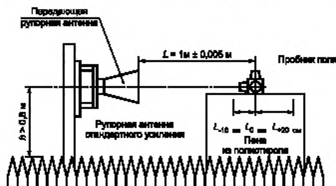
Рисунок I.3 — Испытательная установка для валидации камеры
