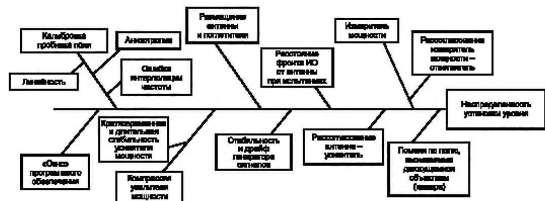
Рисунок J.1 — Пример влияний на установку уровня
