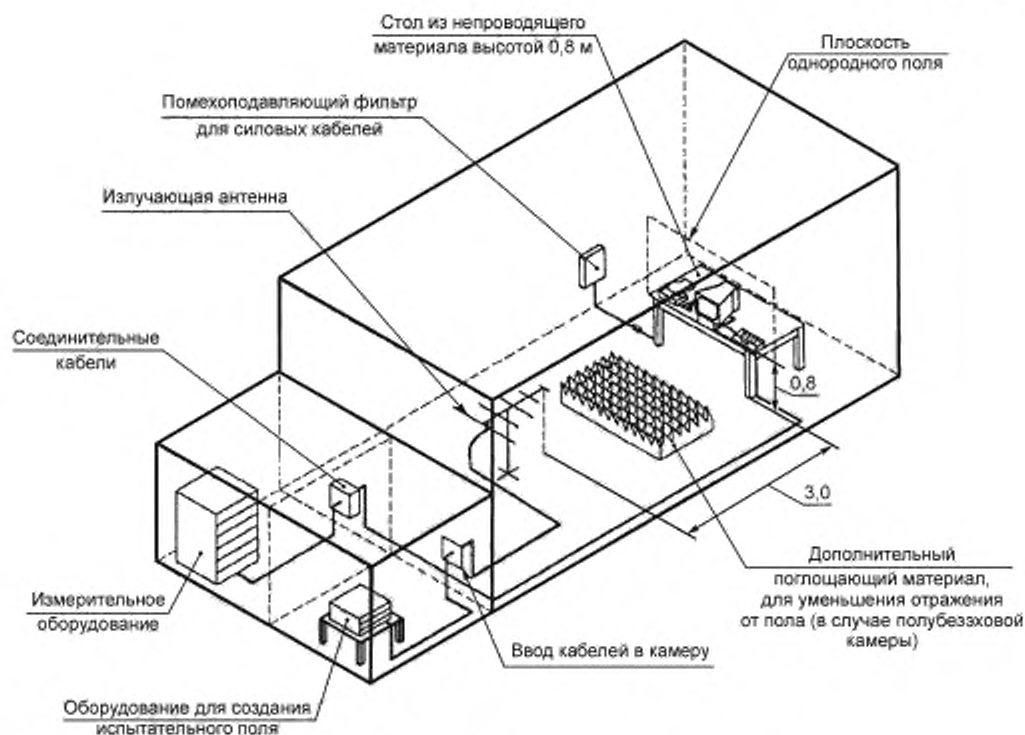
Рисунок 2 — Пример пригодной испытательной установки
