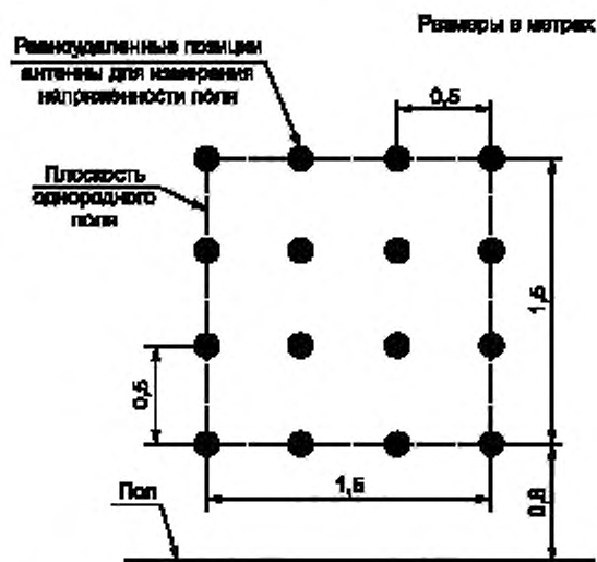
Рисунок 4 — Калибровка поля; размеры плоскости однородного поля
