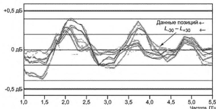
Рисунок I.8 — Пример данных альтернативной валидации камеры
