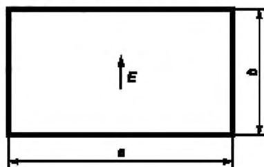
Рисунок 1.11 — Поперечное сечение волноводной камеры
