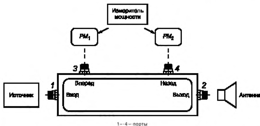
Рисунок 1.2 — Установка для измерения мощности, поступающей к передающему устройству
