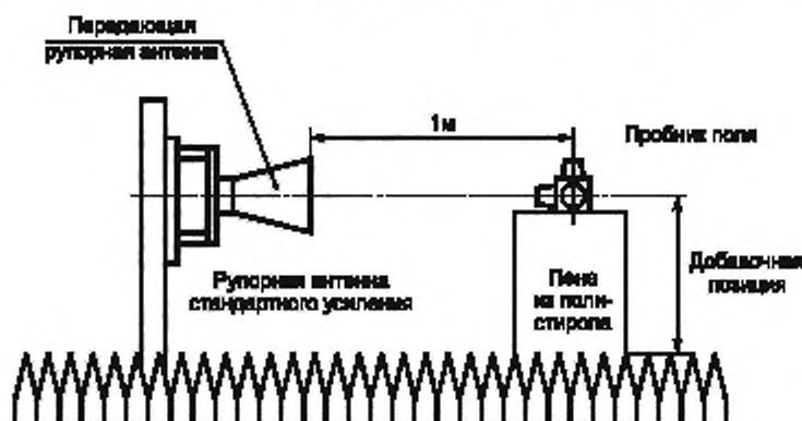
Рисунок I.6 — Пример испытательного расположения антенны и пробника
