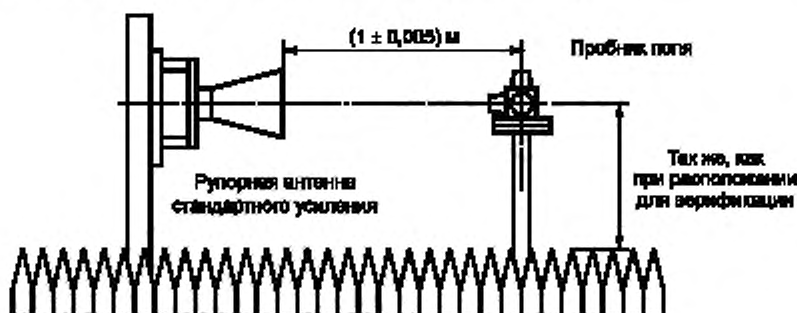
Рисунок 1.9 — Расположение пробника поля при калибровке
