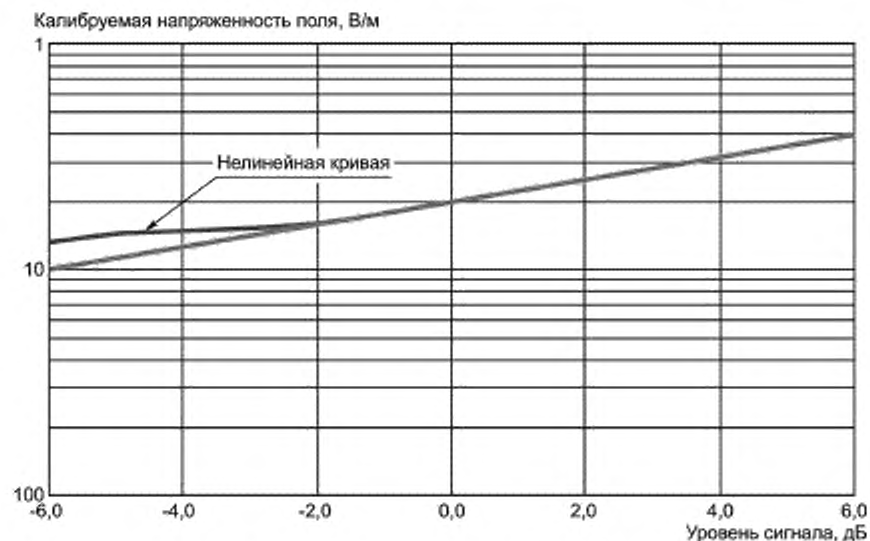
Рисунок I.1 — Пример линейности пробника
