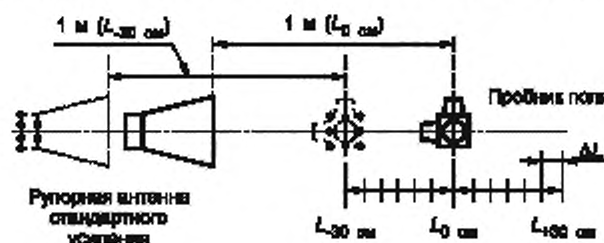
Рисунок I.7 — Испытательная установка для валидации камеры
