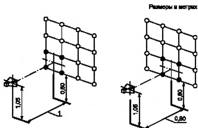
Рисунок Н.2 — Пример последовательного облучения окон
