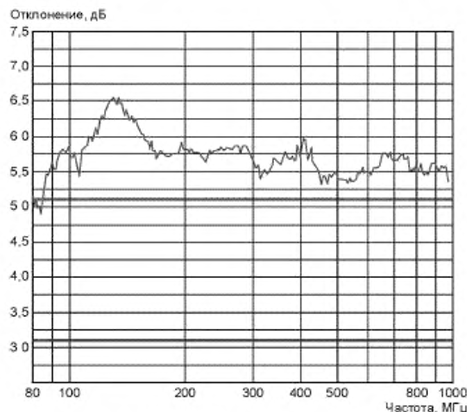
Рисунок 2 (IS 1) — Отклонения по шагу j-3 для полупроводникового усилителя (IS 1, 2008)
