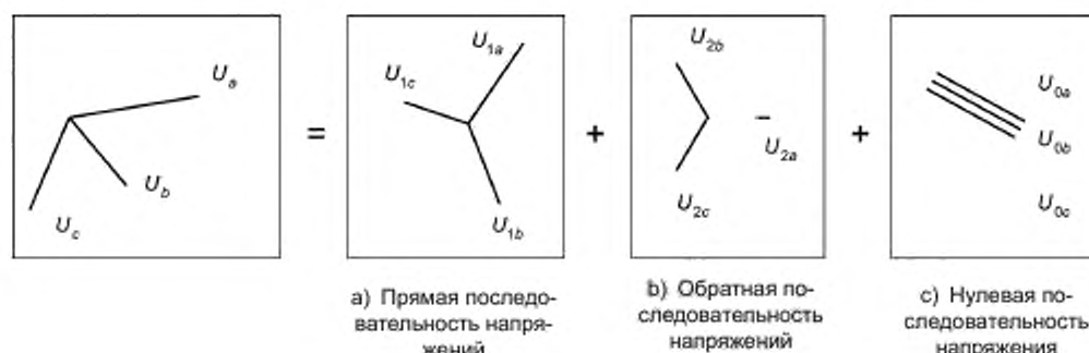
Рисунок А.2 — Составляющие несимметричных векторов на рисунке А.1
