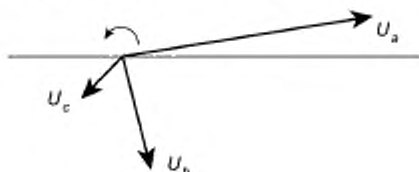
Рисунок А.1 — Несимметричные векторы напряжения
