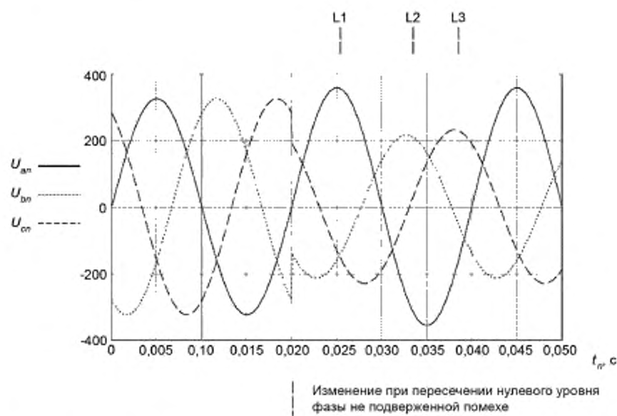
Рисунок 1 — Пример несимметричного трехфазного напряжения питания (испытание 3)
