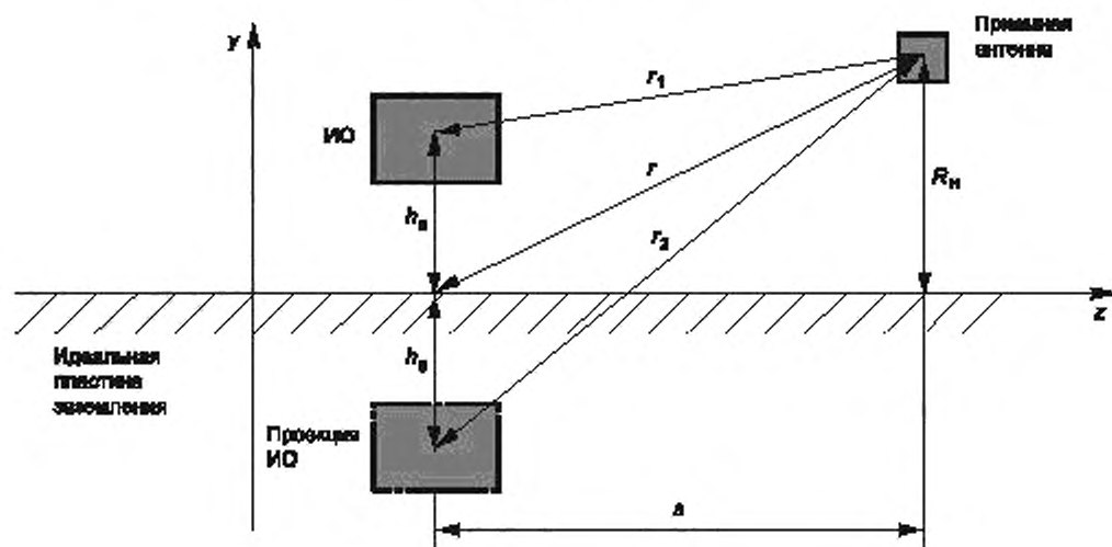
Рисунок A.4 Лист 2
