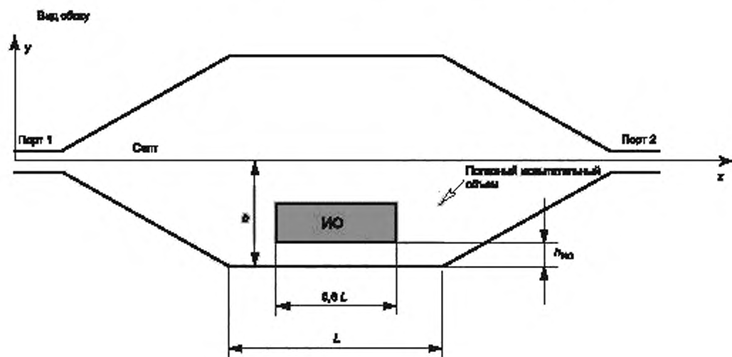
Рисунок A.6a — Вид сбоку
