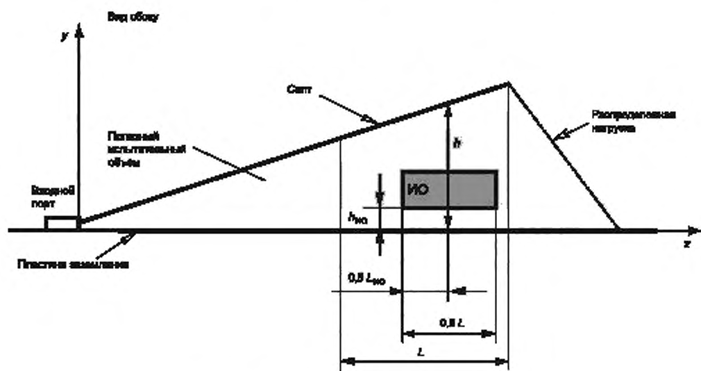
Рисунок А.8а — Вид сбоку (однопортовый волновод)
