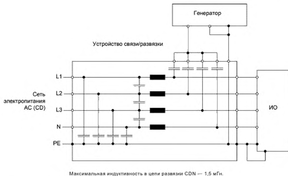
Рисунок 6b — Испытательная установка, снабженная специальными заземляющими проводниками
