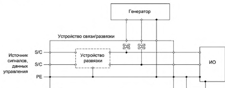
Рисунок 11b — Испытательная установка, снабженная специальными заземляющими проводниками
