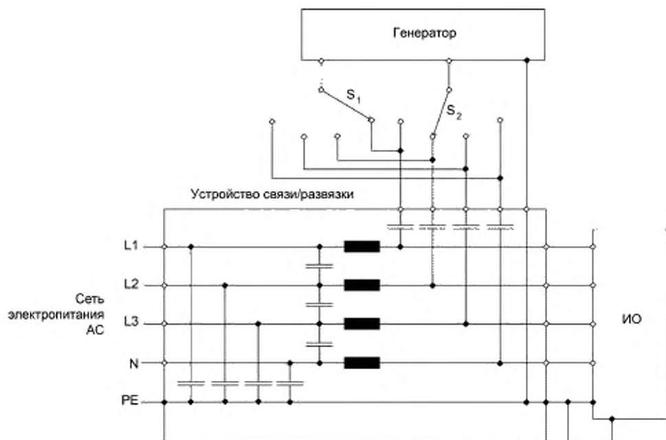
Рисунок 10b — Испытательная установка, снабженная специальными заземляющими проводниками
