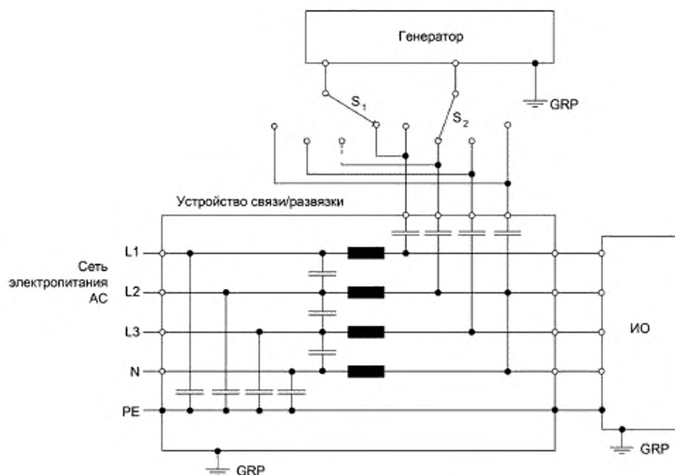
Рисунок 10a — Испытательная установка, снабженная опорной пластиной заземления (GRP)
