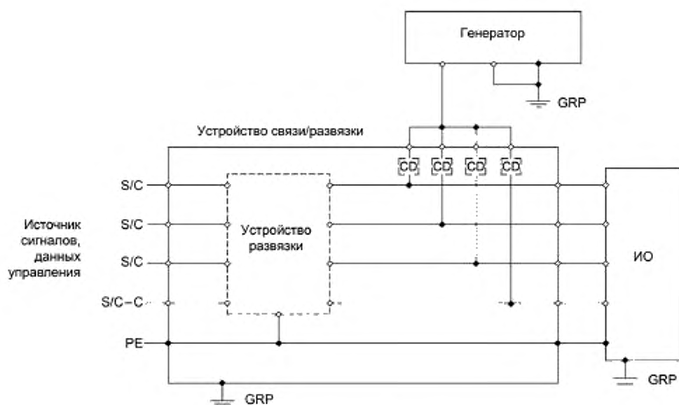
Рисунок 8a — Испытательная установка, снабженная опорной пластиной заземления (GRP)
