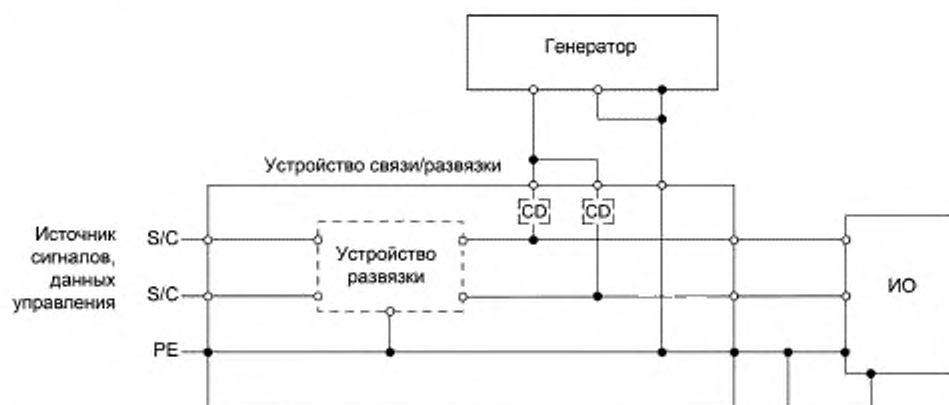
Рисунок 7b — Испытательная установка, снабженная специальными заземляющими проводниками
