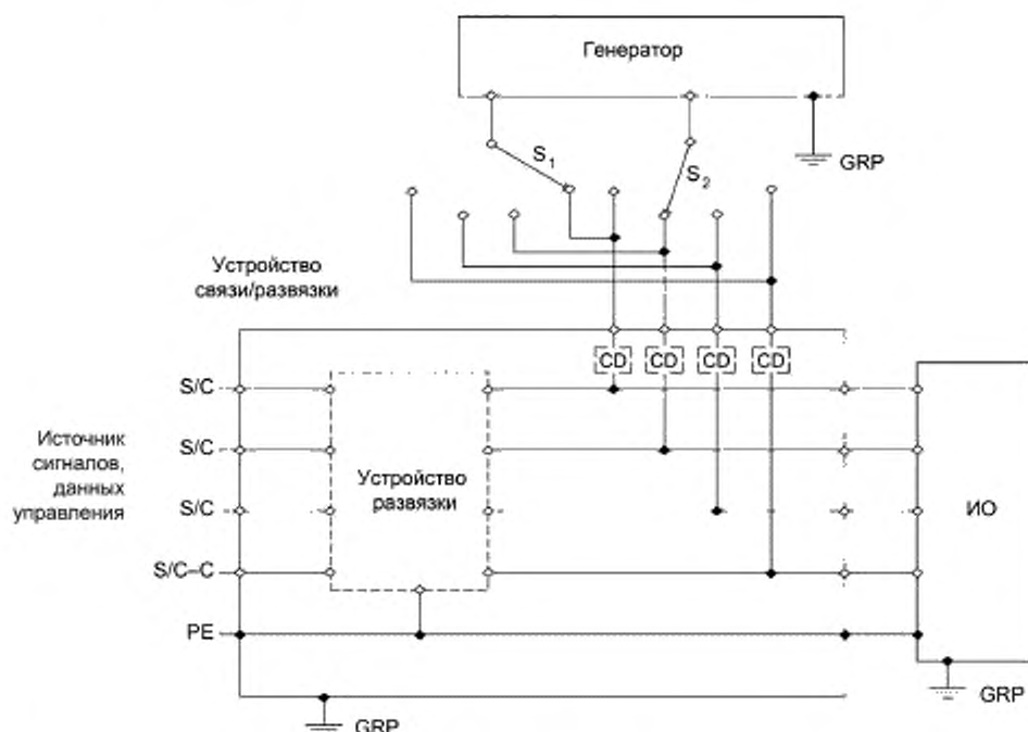
Рисунок 12a — Испытательная установка, снабженная опорной пластиной заземления (GRP)
