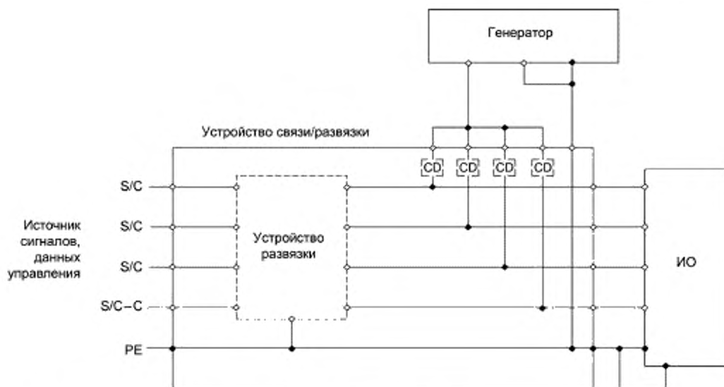
Рисунок 8b — Испытательная установка, снабженная специальными заземляющими проводниками
