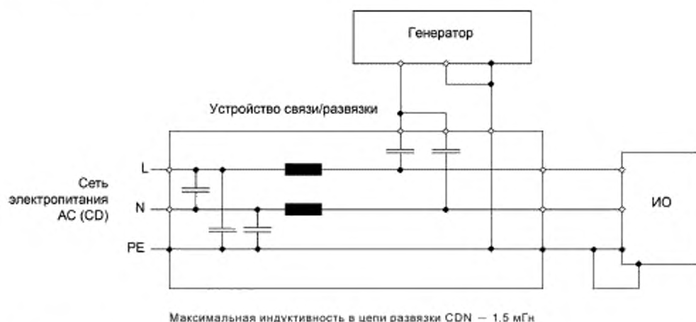
Рисунок 5b — Испытательная установка, снабженная специальными заземляющими проводниками
