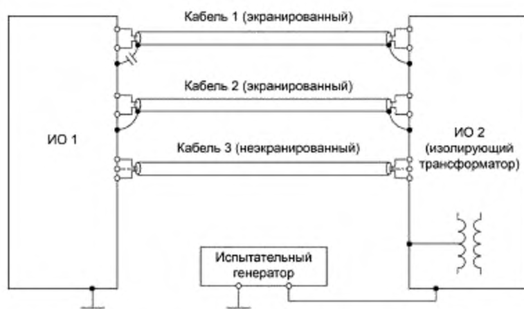
Рисунок 13 — Испытания системы, имеющей порты связи с широкополосными рабочими сигналами (выход генератора заземлен)
