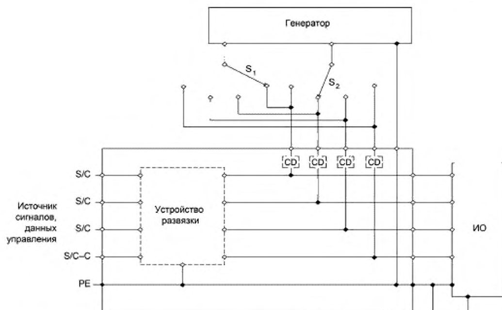
Рисунок 12b — Испытательная установка, снабженная специальными заземляющими проводниками
