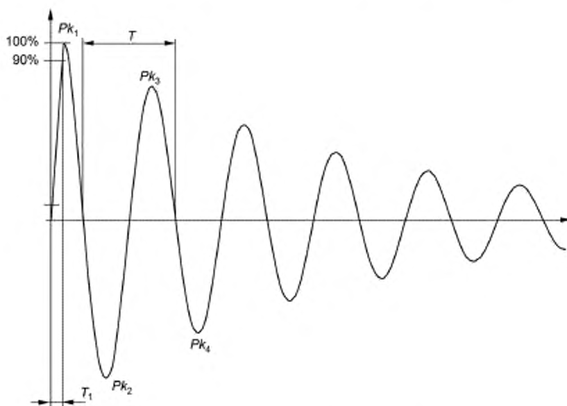
Рисунок 1 — Форма затухающей колебательной волны (напряжение холостого хода)
