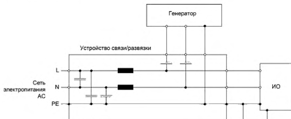
Рисунок 9b — Испытательная установка, снабженная специальными заземляющими проводниками
