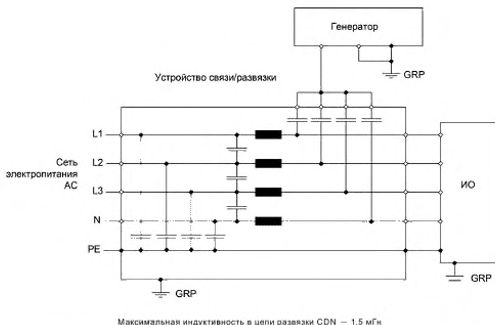
Рисунок 6a — Испытательная установка, снабженная опорной пластиной заземления (GRP)
