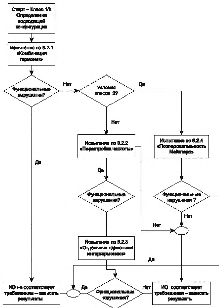
Рисунок 1а — Алгоритм проведения испытаний для классов электромагнитной обстановки 1 и 2
