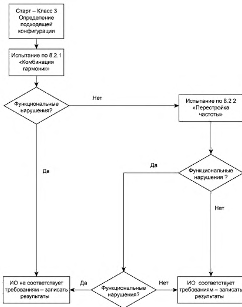
Рисунок 1b — Алгоритм проведения испытаний для класса электромагнитной обстановки 3
