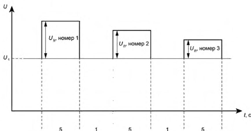
Рисунок 4 — Испытательная последовательность для отдельных гармоник
