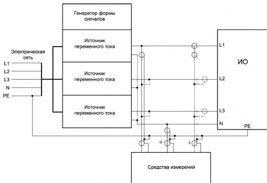
Рисунок 3 — Пример испытательной установки для трехфазной сети
