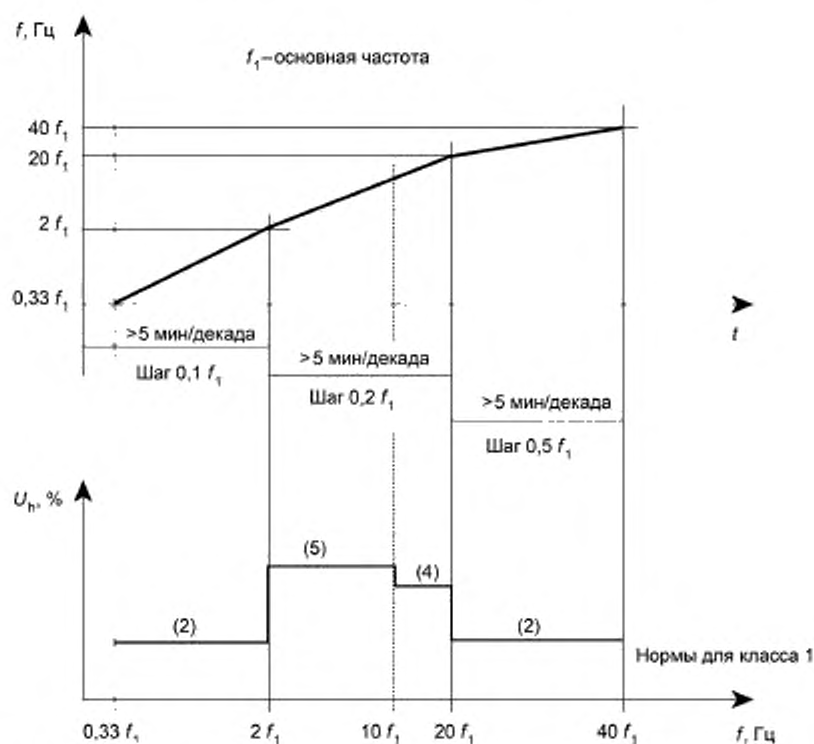
Рисунок 4 — Испытательная последовательность для отдельных гармоник
