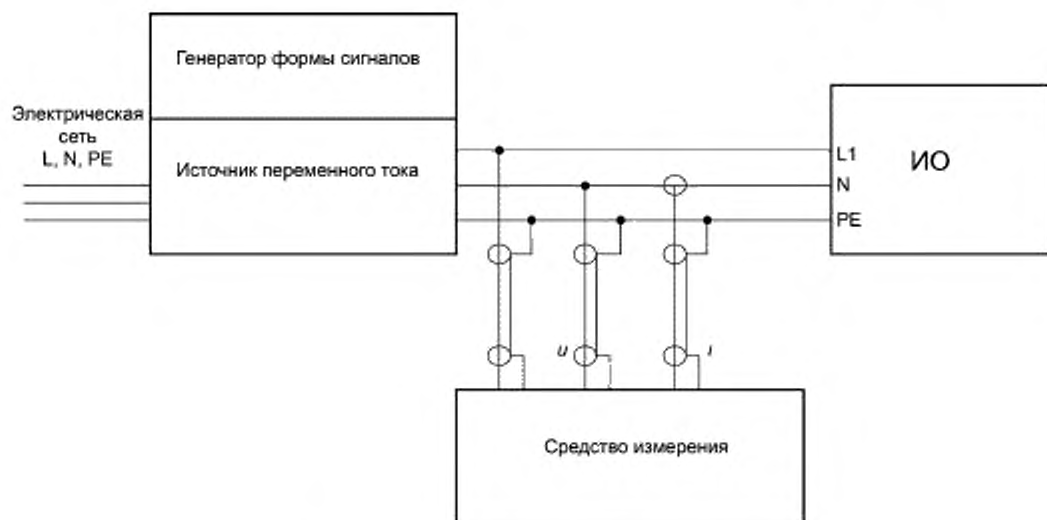
Рисунок 2 — Пример испытательной установки для однофазной сети
