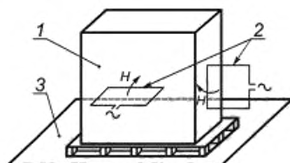
1 — ИО; 2 — индукционная катушка; 3 — эталонная пластина заземления
