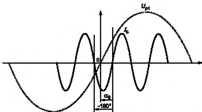
Рисунок 2 — Определение угла фазового сдвига гармонической составляющей тока 5-го порядка I_5 относительно основной составляющей фазного напряжения U_{p1} ( I_5 отстает от U_{p1} , \alpha_5 < 0 )
