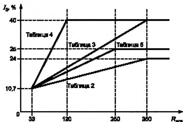
Рисунок В.1 — Зависимость норм гармонической составляющей тока 5-го порядка от R_{sce}
