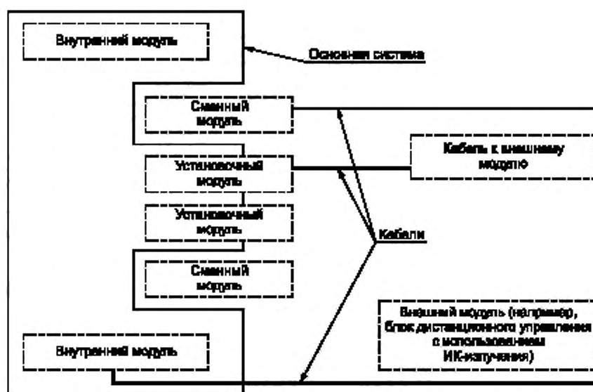
Рисунок 2 — Пример основной системы с модулями разных типов
