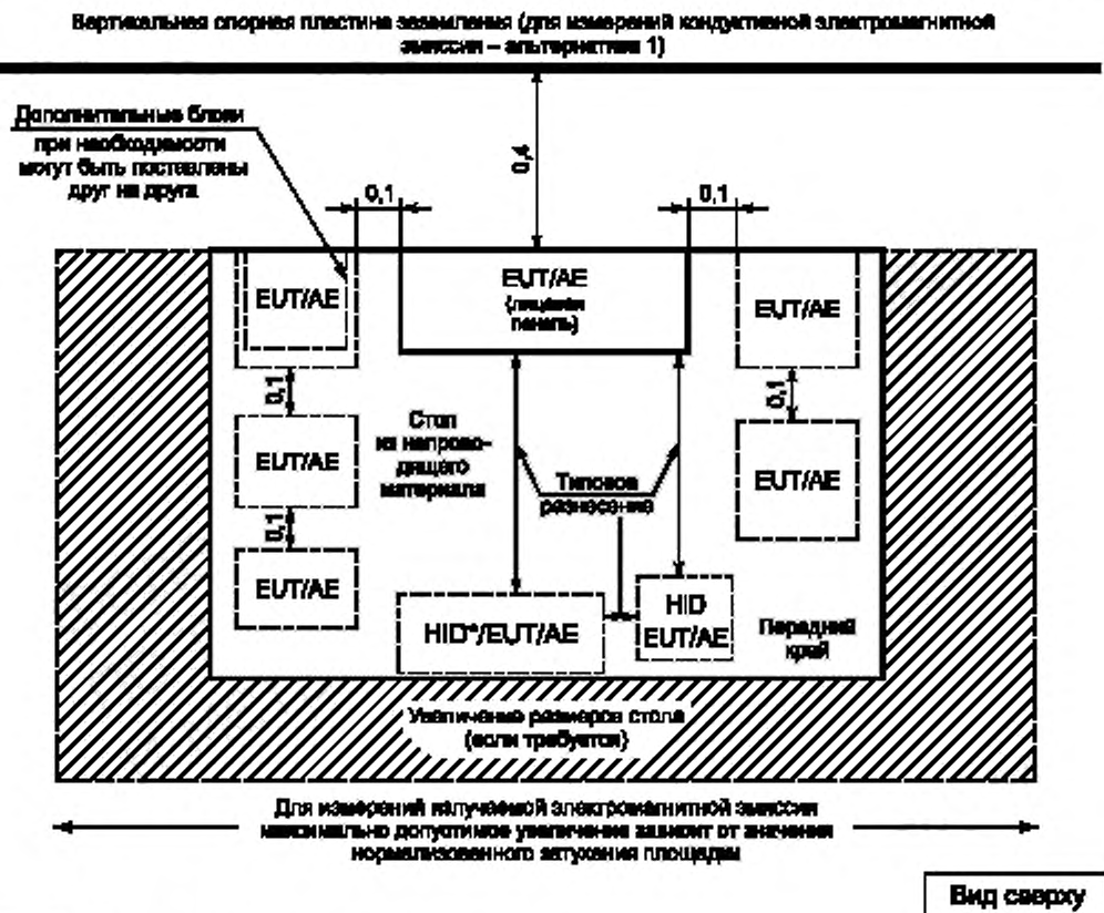
Рисунок D.1 — Пример схемы измерения настольного EUT (кондуктивная и излучаемая электромагнитная эмиссия) (вид сверху)
