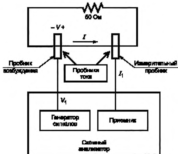
Рисунок С.6 — Калибровочная оправка
