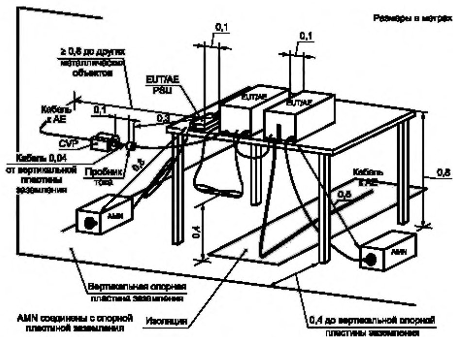
Рисунок D.4 — Пример схемы измерения настольного EUT при измерении в соответствии с C.4.1.6.4
