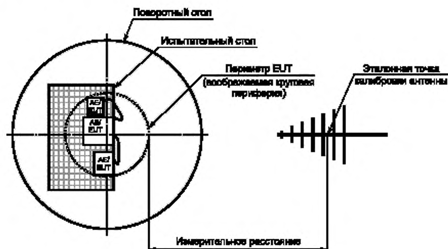
Рисунок С.1 — Измерительное расстояние
