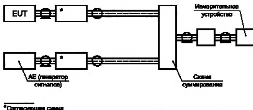
Рисунок С.7 — Компонировка схемы измерения напряжения эмиссии на портах тюнера ТВ/ЧМ-приемников
