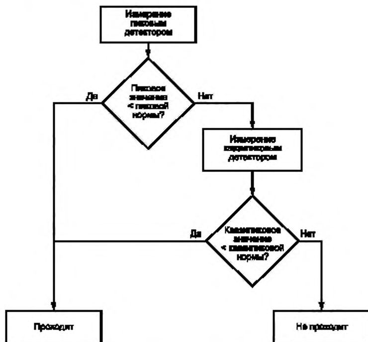
Рисунок С.5 — Алгоритм принятия решения при использовании разных детекторов с нормами в квазипологовых значениях
