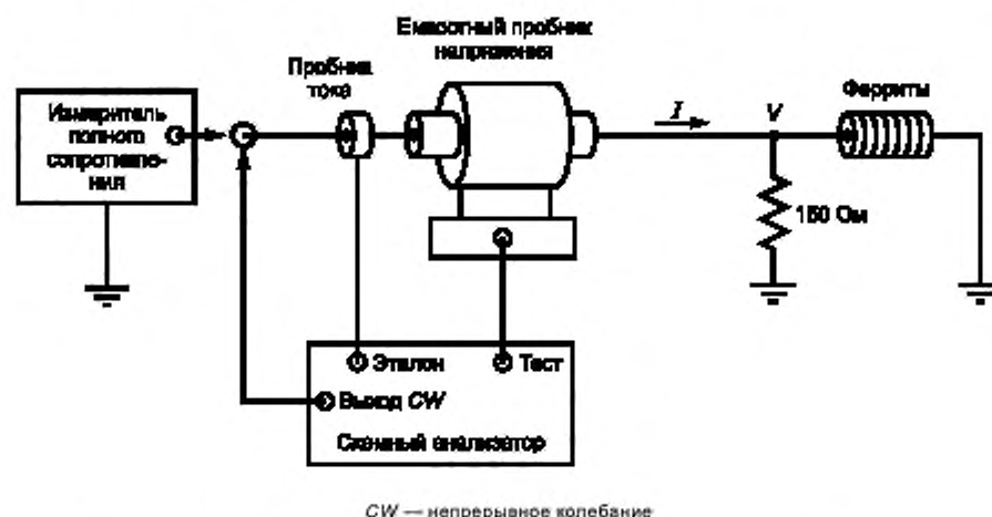
Рисунок G.15 — Основная измерительная установка для измерения суммарного полного сопротивления 150 Ом и ферритов
