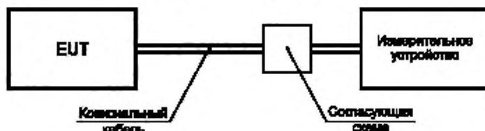
Рисунок С.8 — Компонировка схемы измерения полезного сигнала и напряжения электромагнитной эмиссии на выходном порте ВЧ-модулятора EUT
