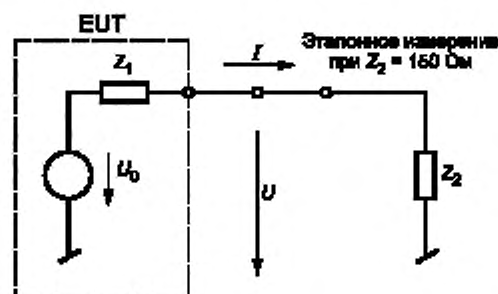
Рисунок G.12 — Базовая схема при рассмотрении норм с указанным общим несимметричным полным сопротивлением 150 Ом
