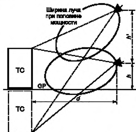
GP — плоскость земли (плоская земля); d = 3 м, h = 1 м, h' = 2,5 м, высота ТС = 1,5 м
