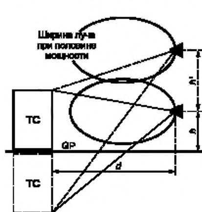
GP — плоскость земли (плоская земля); d = 3 м, h = 1 м, h' = 2,5 м, высота ТС = 1,5 м
