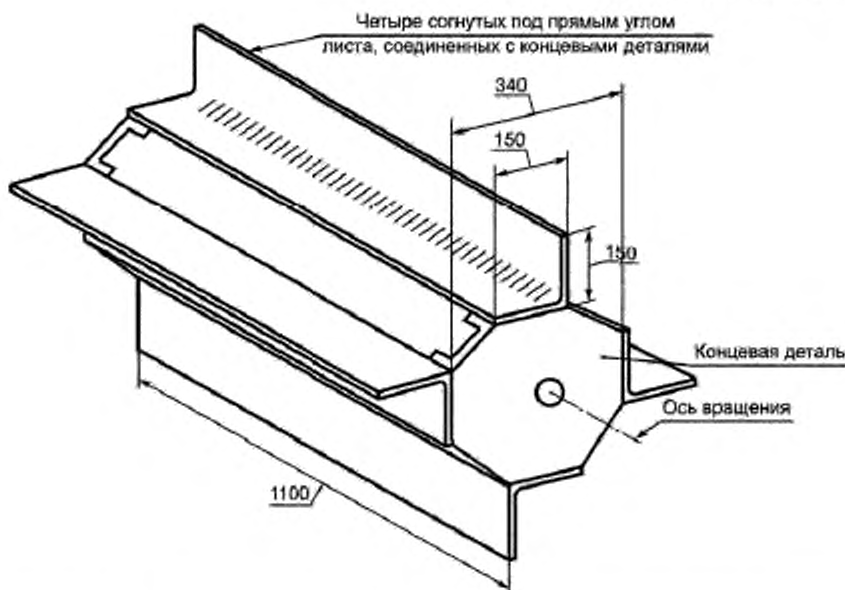
Рисунок 16 — Пример типичного рассеивающего устройства с вращающимися лопатками
