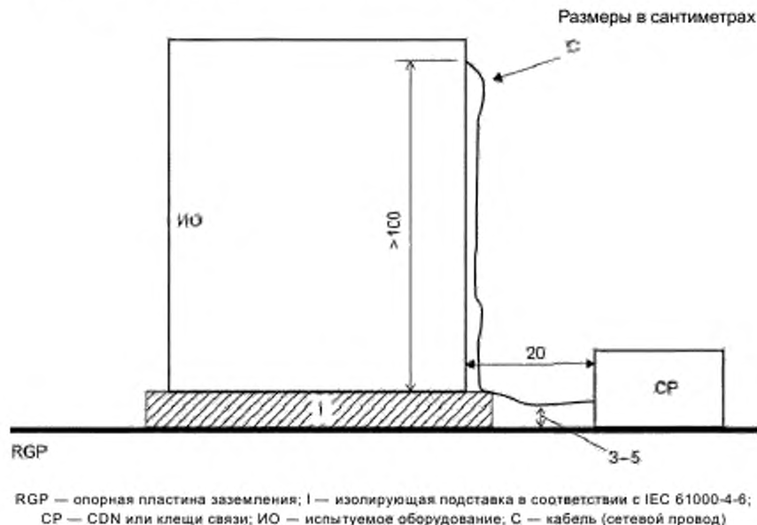
Рисунок 2 — Пример испытательной установки для ИО больших размеров (например, холодильников) с кабелем, отходящим от ИО на высоте более 1 м над полом
