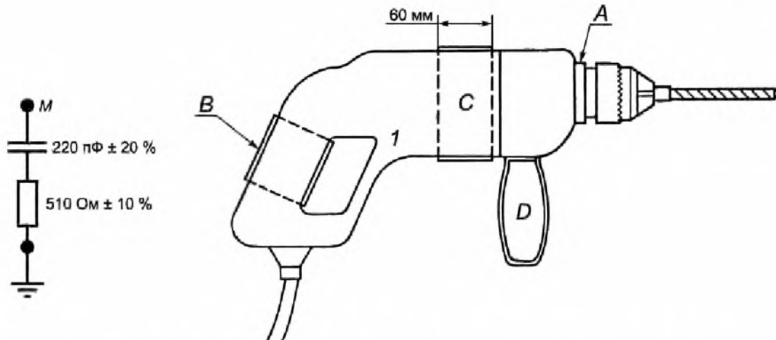
Рисунок 8a) — Элемент RC
