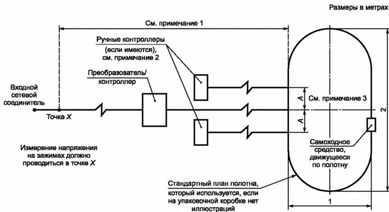
Рисунок 6 — Схема измерений напряжения помех, создаваемых на зажимах устройств питания электрических ограждений (см. 7.3.7.2)
