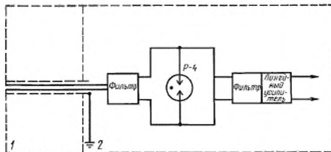
1 — кабельный ввод; 2 — междугородная телефонная станция
