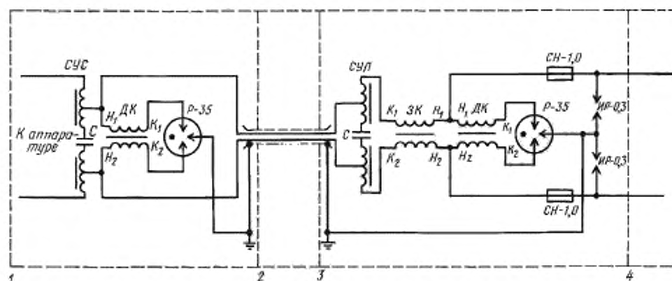
1 — междугородная телефонная станция, УП; 2 — кабельный ввод; 3 — кабельная опора; 4 — стальная или стальной уплотненный цепь воздушной линии
