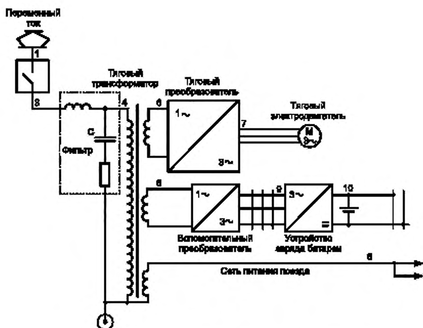
Рисунок А.1 — Система электропитания электровоза переменного тока с тяговыми электродвигателями переменного тока и психометрическим фильтром
