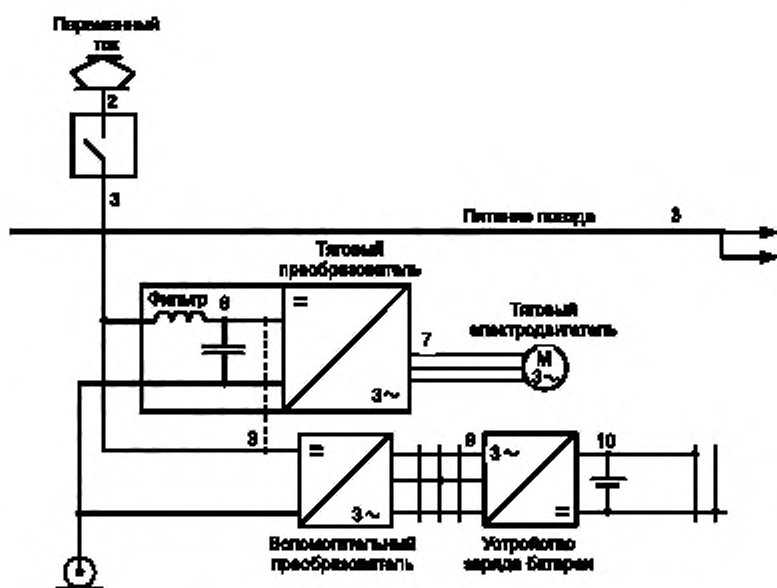
Рисунок А.4 — Система электропитания железнодорожного подвижного состава постоянного тока с тяговыми электродвигателями переменного тока
