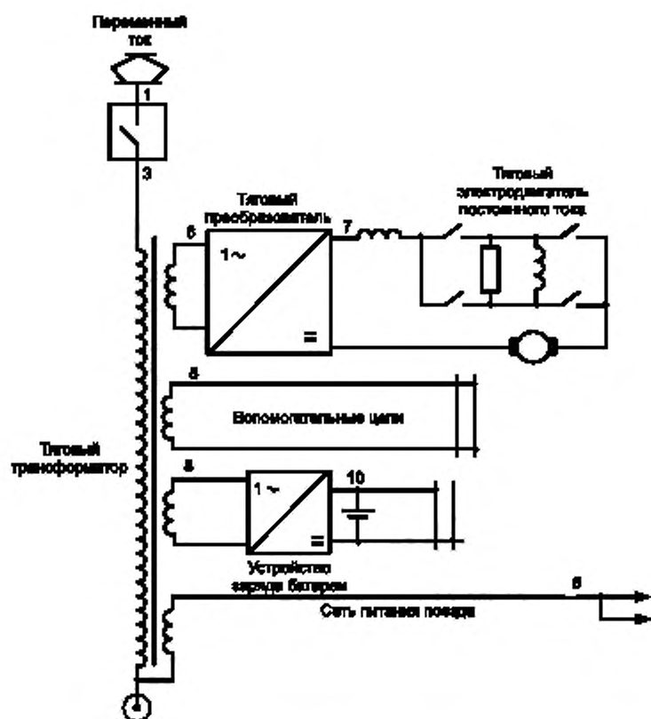
Рисунок А.3 — Система электропитания железнодорожного подвижного состава переменного тока с тяговыми электродвигателями постоянного тока с использованием выпрямительно-инверторного преобразователя
