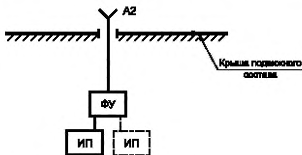
А2 — антенна радиостанции железнодорожной радиосвязи метрового радиочастотного диапазона; ФУ — фильтрующее устройство. ИП — измерительный приемник
