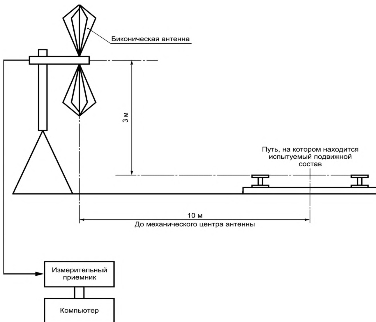
Рисунок 4 — Позиция антенны (вертикальная поляризация) при измерении электрического поля в диапазоне частот от 30 до 300 МГц
