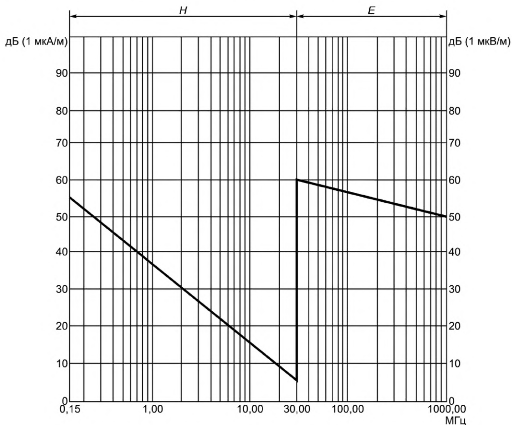
Рисунок 2 — Нормы напряженности поля электромагнитных помех (квазипиковые значения) от тяговых подстанций
