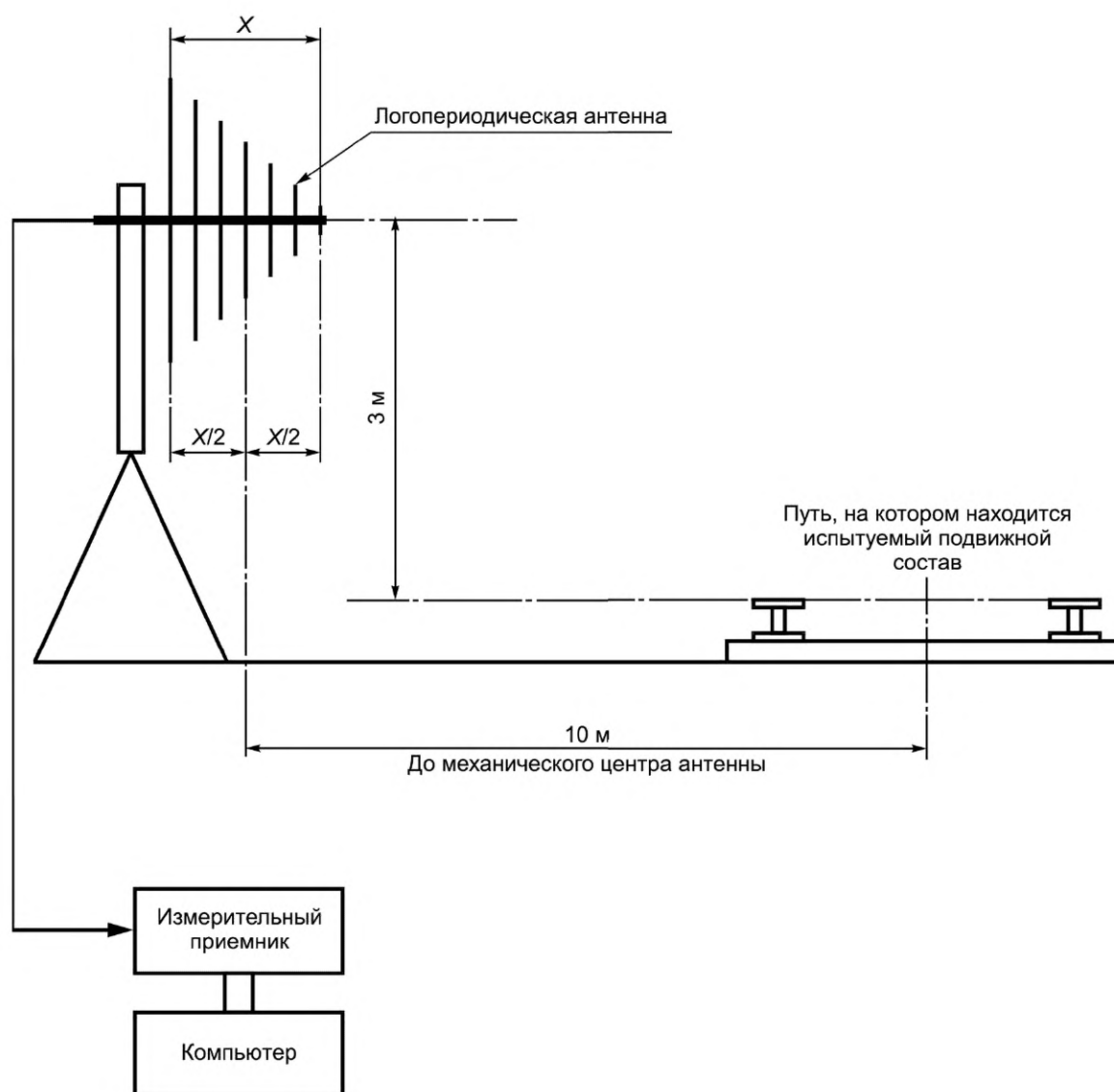
Рисунок 5 — Позиция антенны (вертикальная поляризация) при измерении электрического поля в диапазоне частот от 300 МГц до 1 ГГц
