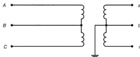
A, B, C — фазы первичной обмотки ТН; a, b, c — фазы основной вторичной обмотки ТН
