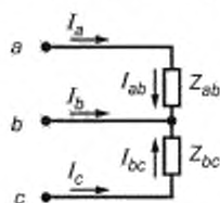
а, b, с — фазы основной вторичной обмотки ТН; I_a, I_b, I_c — фазные токи; I_{ab}, I_{bc} — межфазные токи, Z_{ab}, Z_{bc} — межфазные нагрузки
