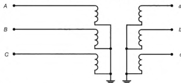
A, B, C — фазы первичной обмотки ТН; a, b, c — фазы основной вторичной обмотки ТН
