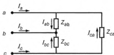
а, b, с — фазы основной вторичной обмотки ТН; I_a, I_b, I_c — фазные токи, I_{ab}, I_{bc}, I_{ca} — межфазные токи; Z_{ab}, Z_{bc}, Z_{ca} — межфазные нагрузки
