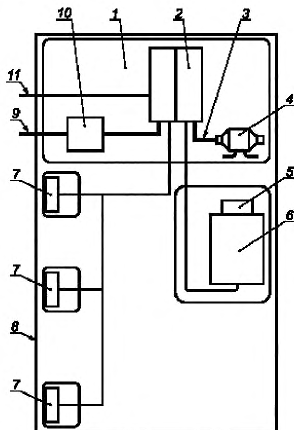
Рисунок 1 — Вариант представления лифта в виде системы (помехозащита)
