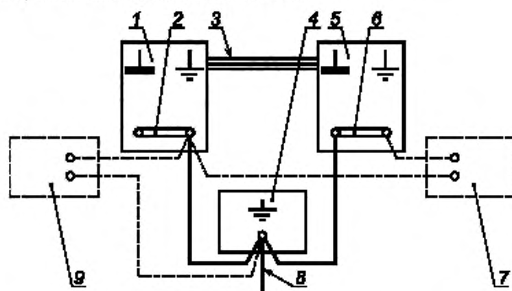
1 — первая стойка испытуемого ТС АС; 2, 6 — перемычки между сигнальной и защитной системами заземления в стойке; 3 — линии связи между стойками; 4 — опорный узел заземления ТС АС; 5 — 2-я стойка испытуемого ТС АС; 7 — подключение ИГ к зажимам защитного заземления двух стоек; 8 — цепь связи с физической землей; 9 — подключение ИГ к зажиму защитного заземления стойки и к опорному узлу заземления
