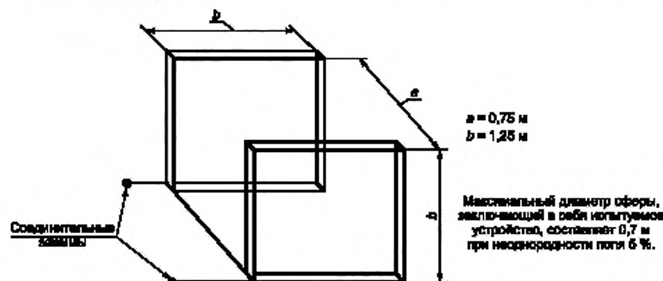
Рисунок A.1 — Конструкция катушки Гельмгольца для однородных полей
