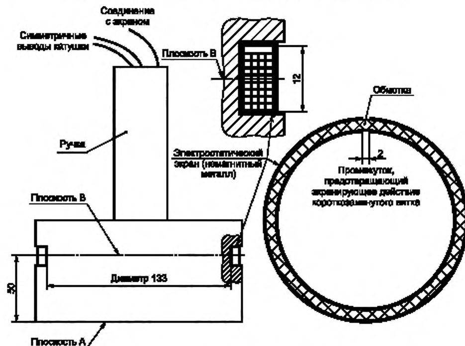
Рисунок A.2 — Конструкция излучающей рамки для неоднородных полей
