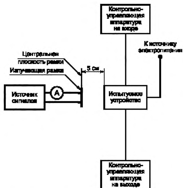
Рисунок А.3 — Типовая схема испытаний для неоднородного магнитного поля в полосе 50 Гц — 10 кГц
