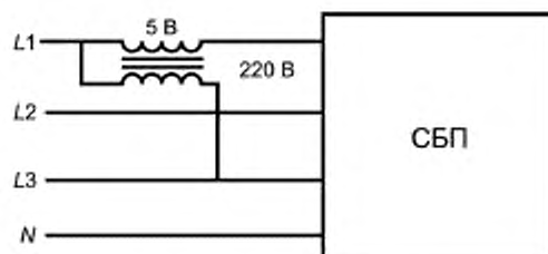
Рисунок D.2 — Фазовая несимметрия
