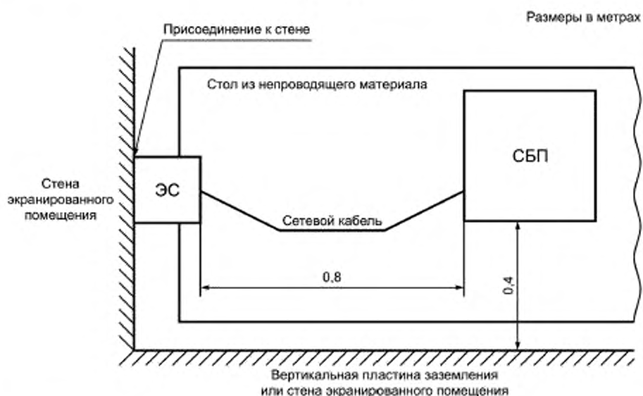
Рисунок А.6 — Размещение испытуемых СБП (настольное оборудование, измерение напряжения ИРП); вид сверху
