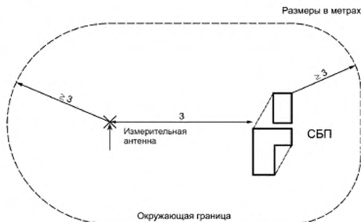
Рисунок А.1 — Схема измерения напряжения ИРП на сетевых зажимах или на выходе СБП
