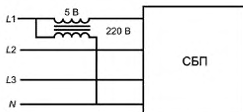
Рисунок D.1 — Амплитудная несимметрия
