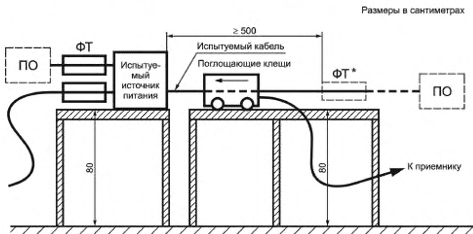
Рисунок 2 — Испытательная установка для измерения мощности промышленных радиопомех
