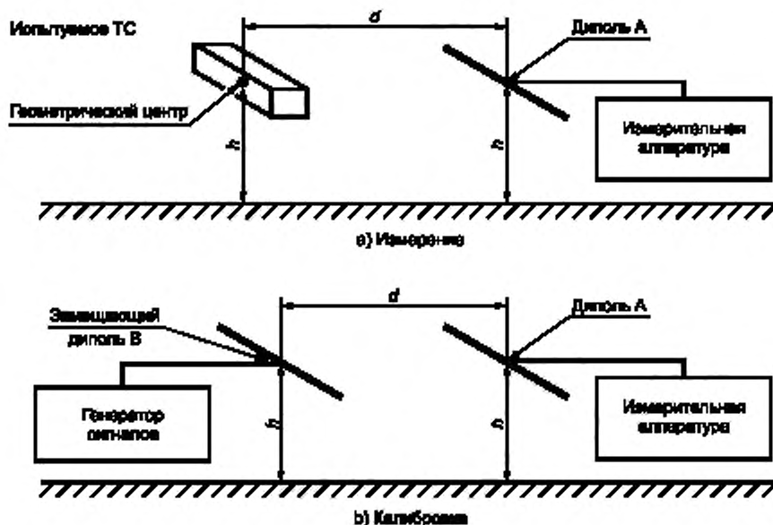
Рисунок 16 — Измерение методом замещения (см. 7.4.1 и 7.4.3)
